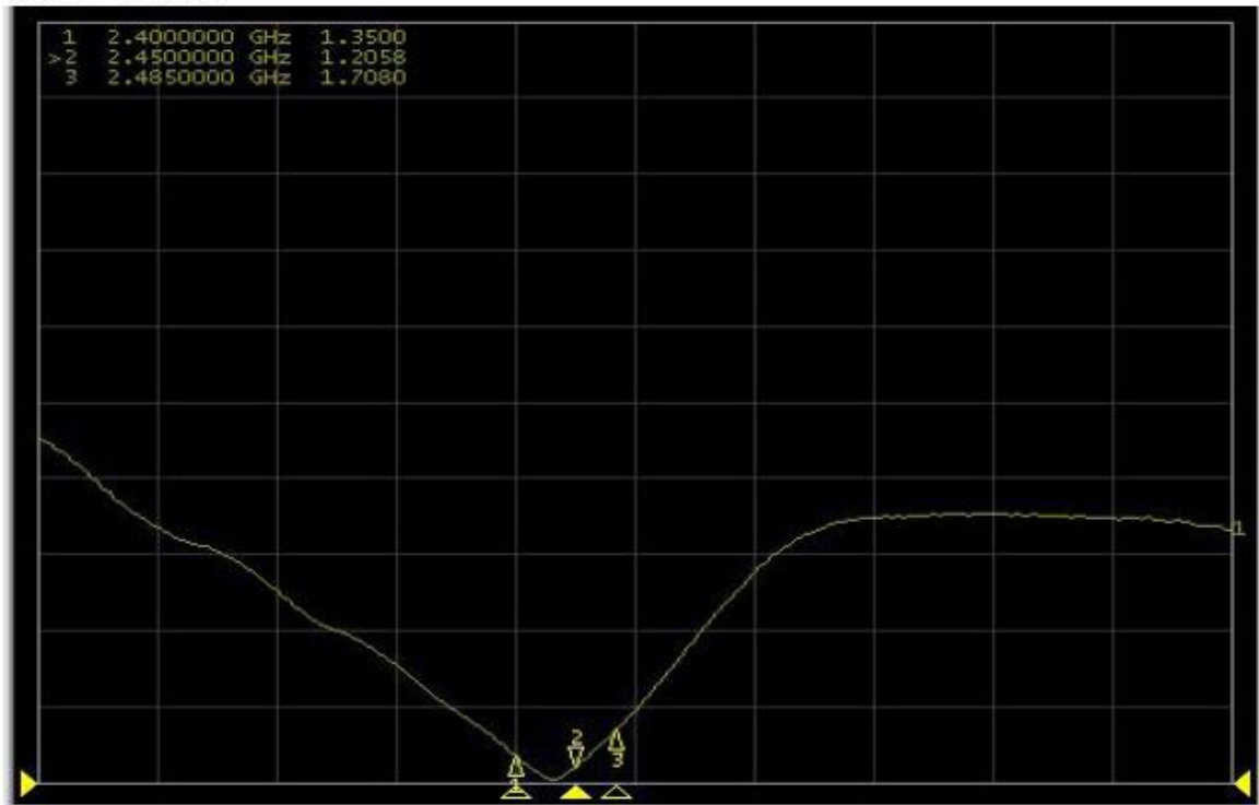
驻波比 (SWR) 图
