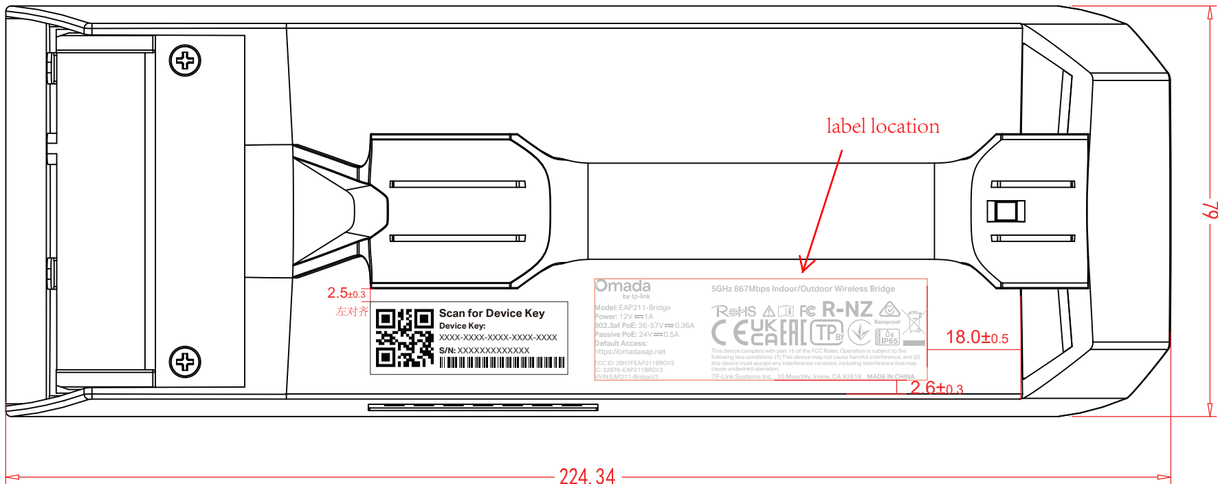
尺寸图
