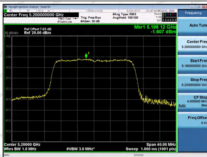
11AX20MIMO-Ant1-5200-PASS
