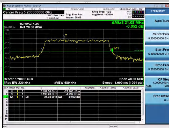
11AX20MIMO-Ant2-5200
