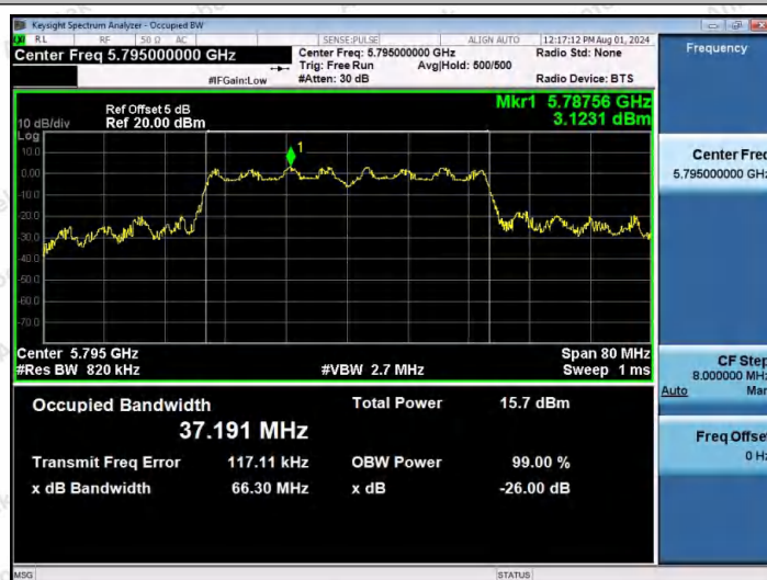
11N40MIMO-Ant2-5795
