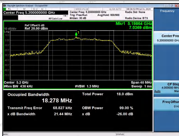
11N20MIMO-Ant1-5200
