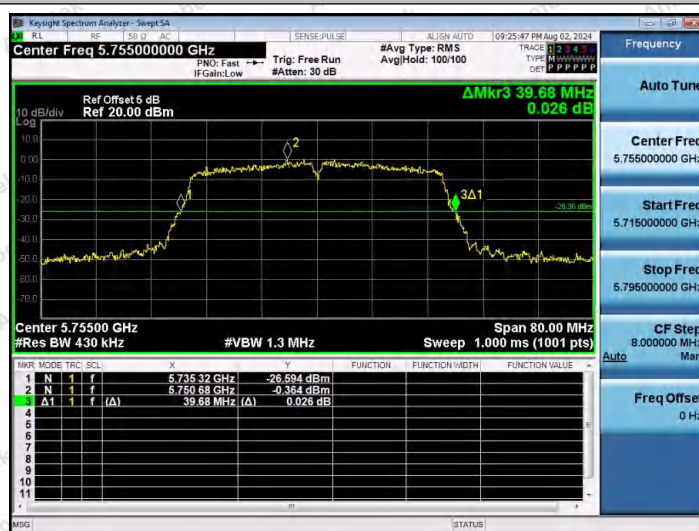
11AX40MIMO-Ant2-5755
