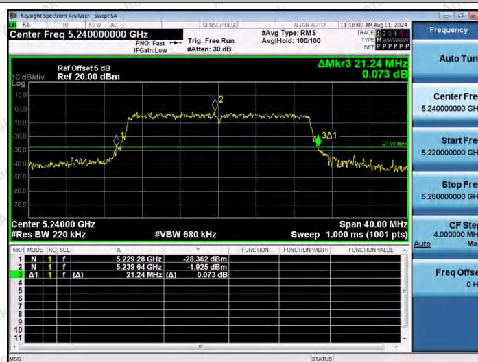
11AX20MIMO-Ant2-5240
