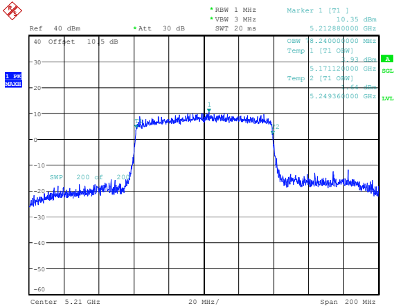
802.11ax80_5210MHz_RU_Full 78.240MHz
