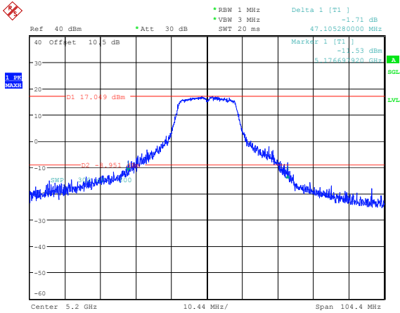
802.11n20_5200MHz 47.105MHz
