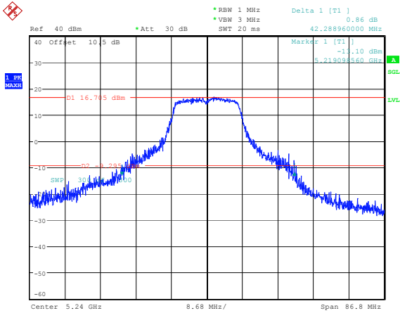
802.11a_5240MHz 42.289MHz
