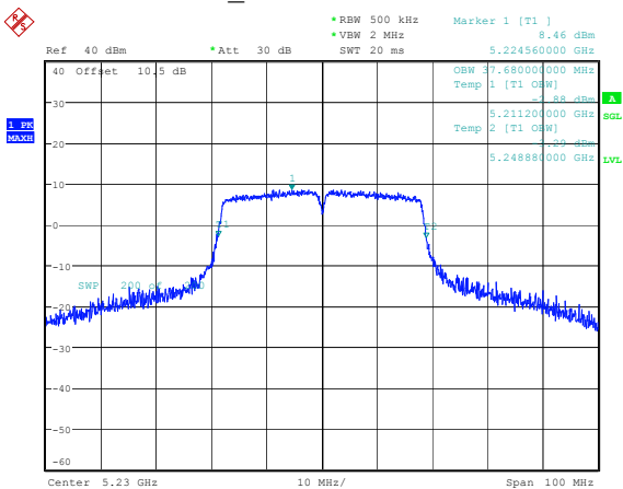
802.11n40_5230MHz 37.680MHz
