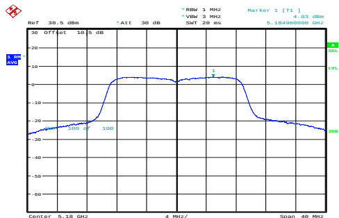
n20_5180MHz_Chain 0 4.03dBm/MHz
