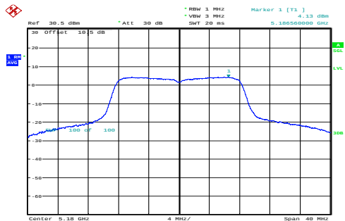
a_5180MHz_Chain 0 4.13dBm/MHz
