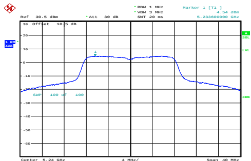
a_5240MHz_Chain 0 4.54dBm/MHz
