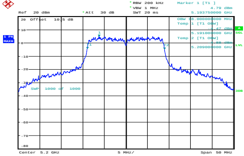
n20_5200MHz_Chain 0 18MHz
