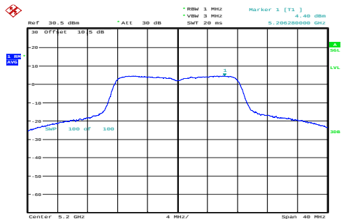
a_5200MHz_Chain 0 4.40dBm/MHz
