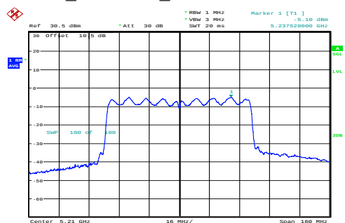
ac80_5210MHz_Chain 0 -5.10dBm/MHz
