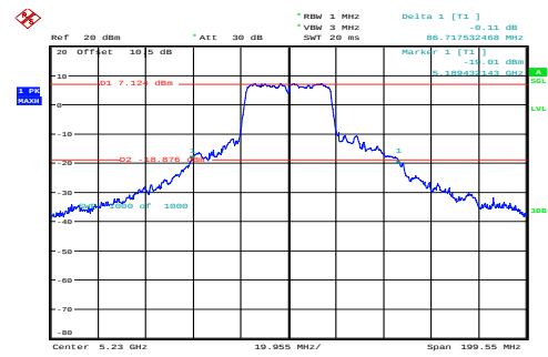
n40_5230MHz_Chain 0 86.718MHz
