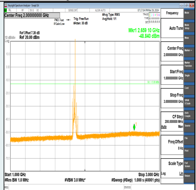
Band2-20MHz-QPSK-18700-1RB#99-1000~3000-PASS
