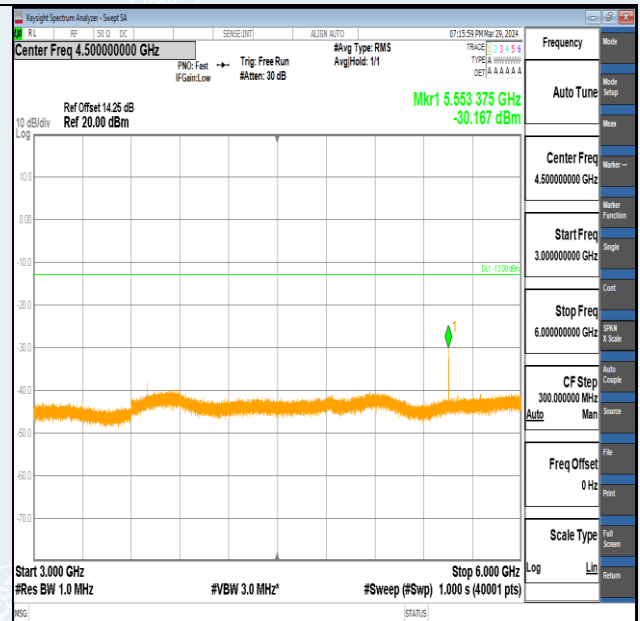
Band2-20MHz-QPSK-18700-1RB#0-3000~6000-PASS
