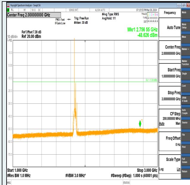
Band2-20MHz-QPSK-18700-1RB#0-1000~3000-PASS
