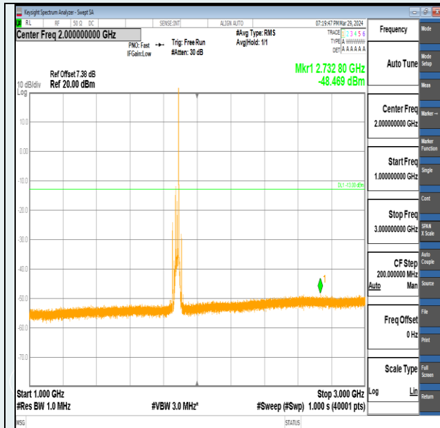
Band2-20MHz-QPSK-18900-1RB#99-1000~3000-PASS
