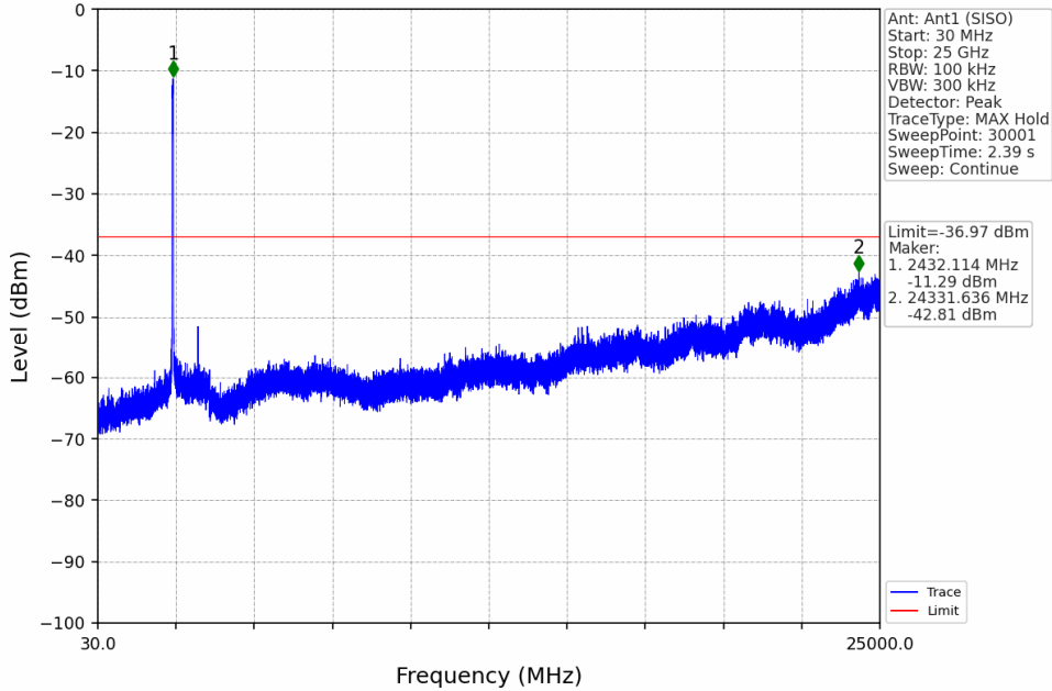
802.11n(HT40)_MCH_2437MHz_Ant1 (SISO)_NTNV
