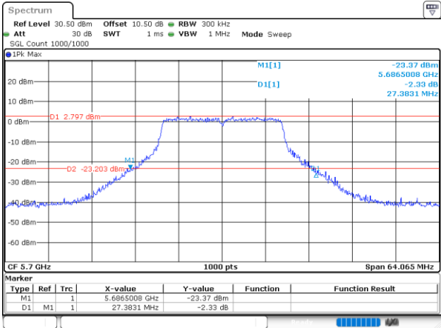
802.11ac20_5700MHz
