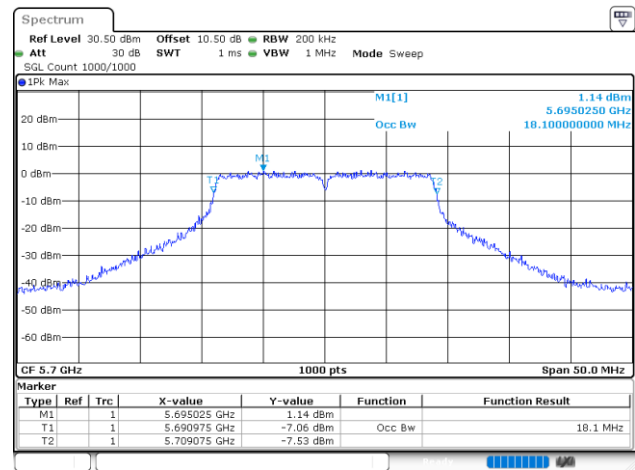
802.11ac20_5700MHz
