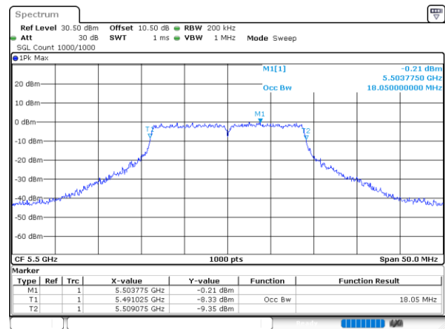
802.11ac20_5500MHz
