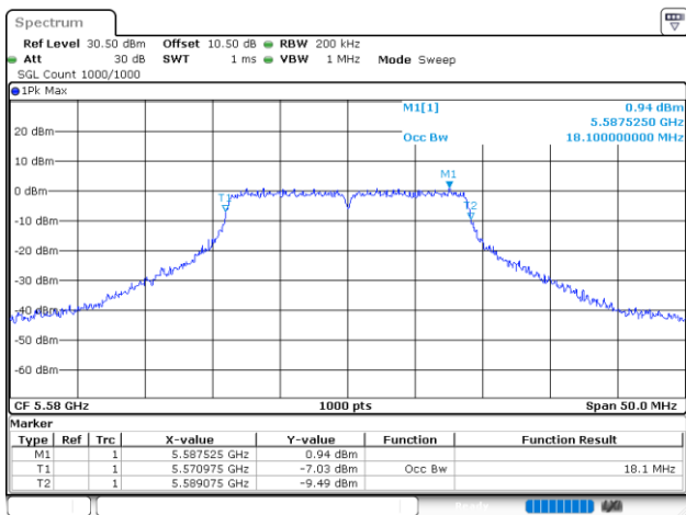
802.11ac20_5580MHz
