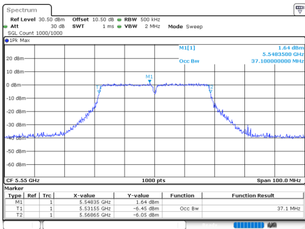
802.11ac40_5550MHz
