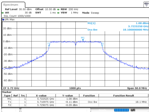
802.11ac20_5720MHz
