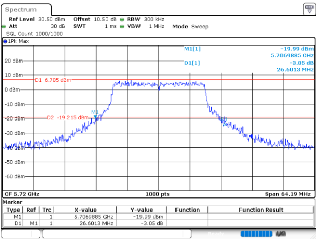
802.11ax20_5720MHz_RU_Full
