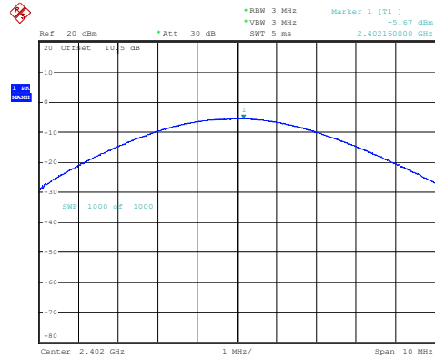
\pi/4 -DQPSK_Low -5.67dBm
