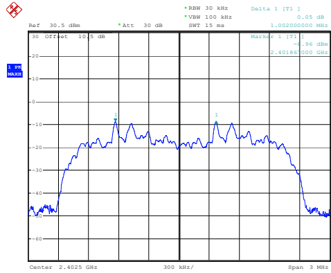
\pi/4 -DQPSK_Low 1.002MHz
