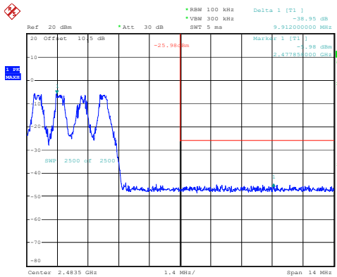
GFSK_Hopping_Upper
