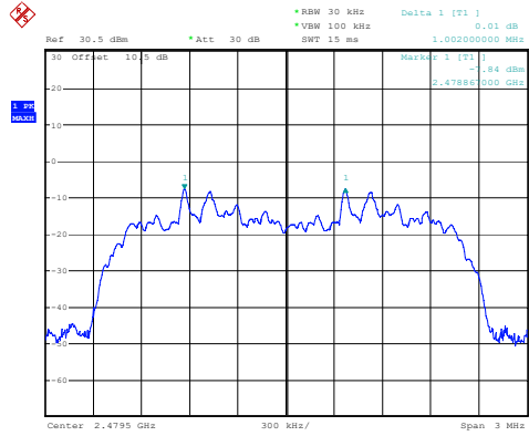
\pi/4 -DQPSK_High 1.002MHz
