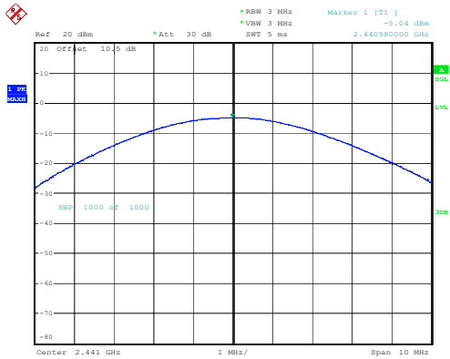
\pi/4 -DQPSK_Middle -5.04dBm
