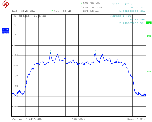
\pi/4 -DQPSK_Middle 1.002MHz
