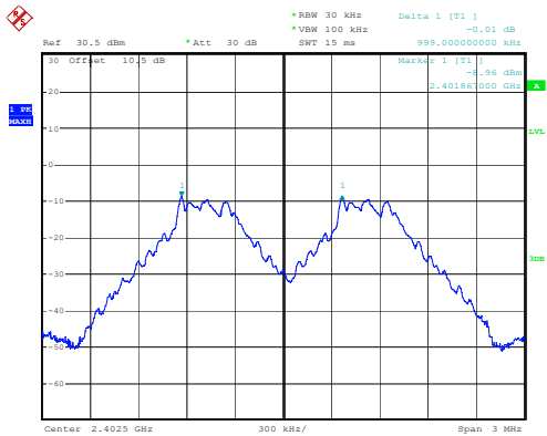
GFSK_Low 0.999MHz
