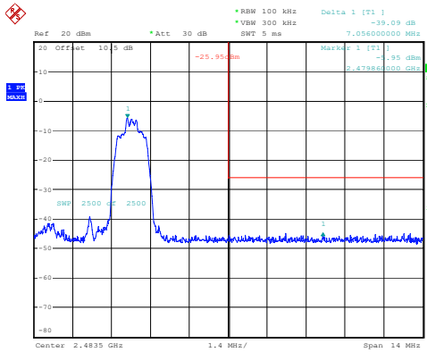
\pi/4 -DQPSK_High
