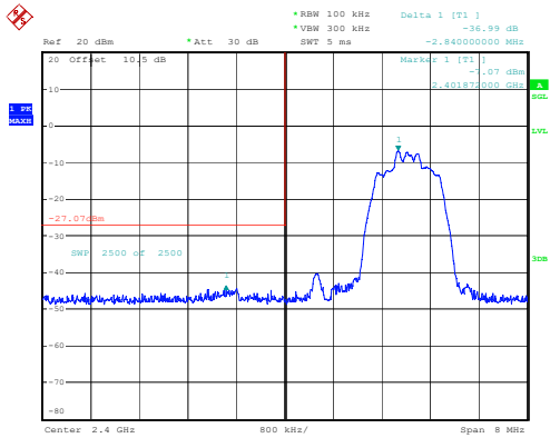
\pi/4 -DQPSK_Low
