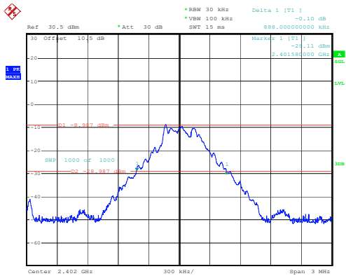
GFSK_Low 0.888MHz
