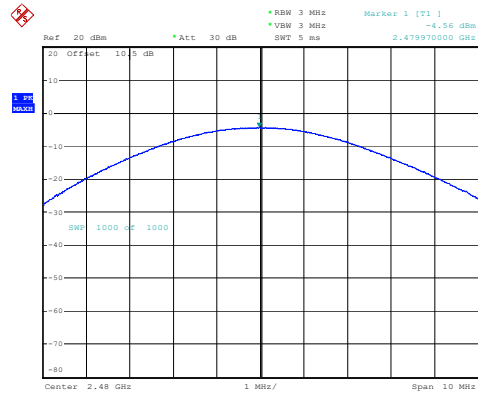
\pi/4 -DQPSK_High -4.56dBm
