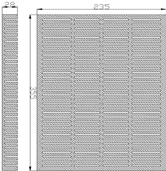
侧面图
