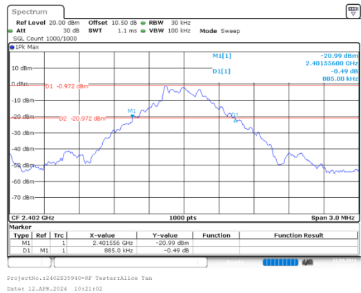
GFSK_Low_DH1
