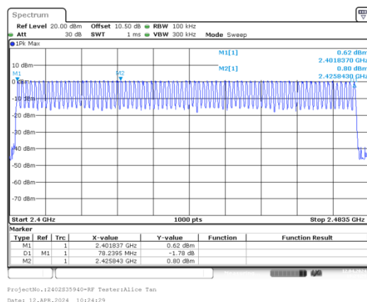
GFSK_Hopping_DH1
