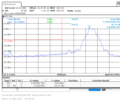
GFSK_Low_DH1
