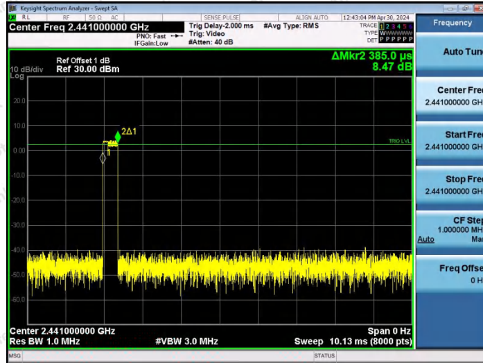
3DH1-Ant0-Hop-PASS
