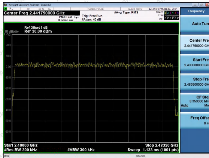
2DH5-Ant0-Hop-PASS
