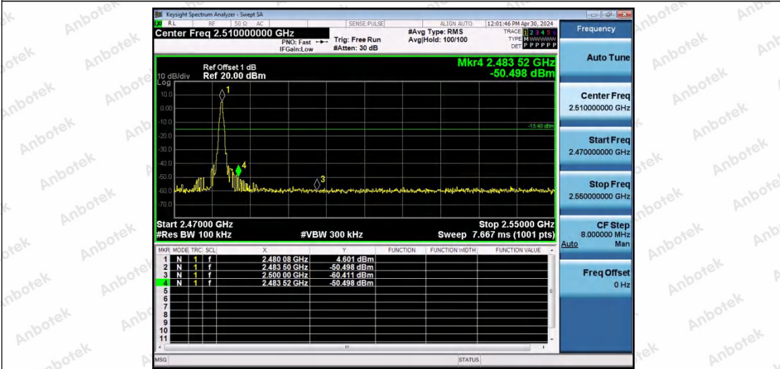
DH5-Ant0-2480-PASS
