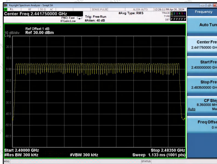
DH5-Ant0-Hop-PASS
