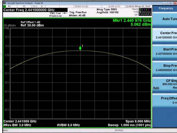
DH5-Ant0-2441-PASS
