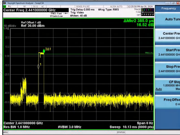
2DH1-Ant0-Hop-PASS
