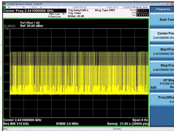
2DH1-Ant0-Hop-PASS
