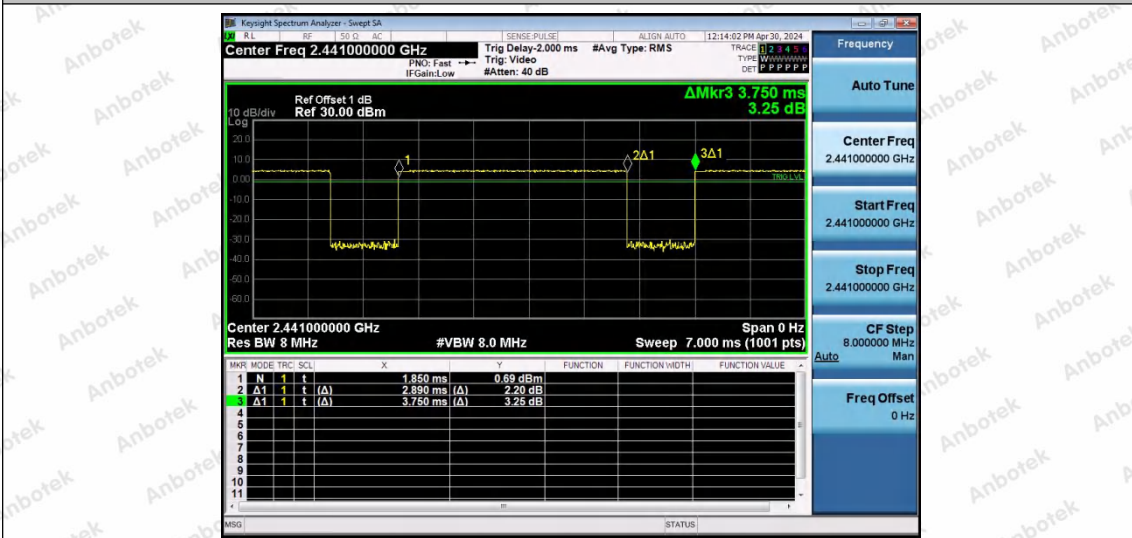
NTNV-3DH5-Ant0-2441
