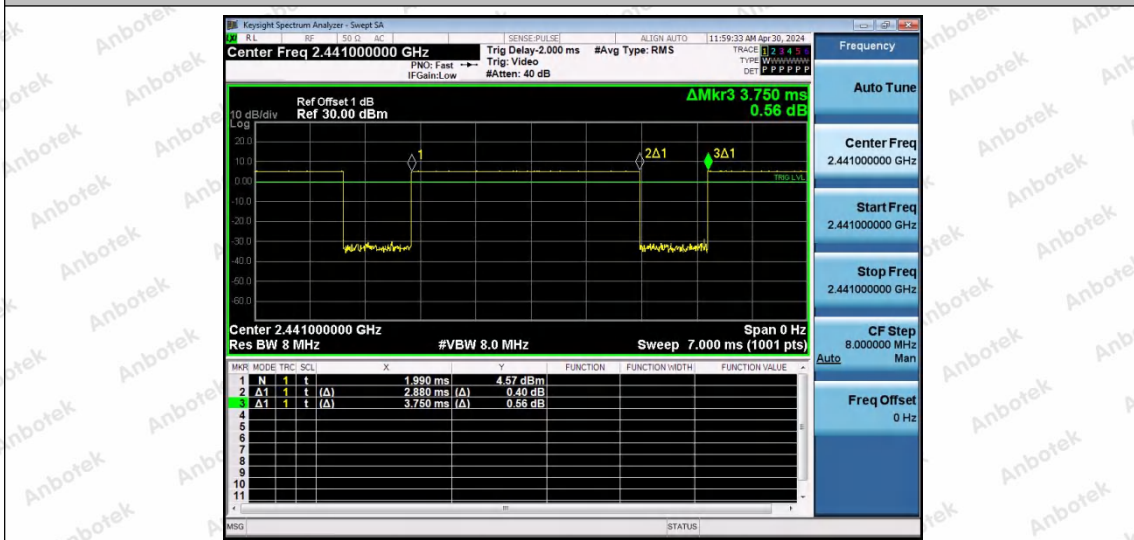
NTNV-DH5-Ant0-2441
