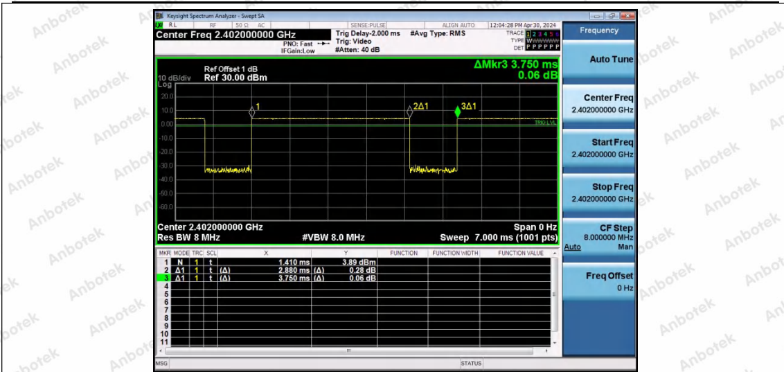
NTNV-2DH5-Ant0-2402
