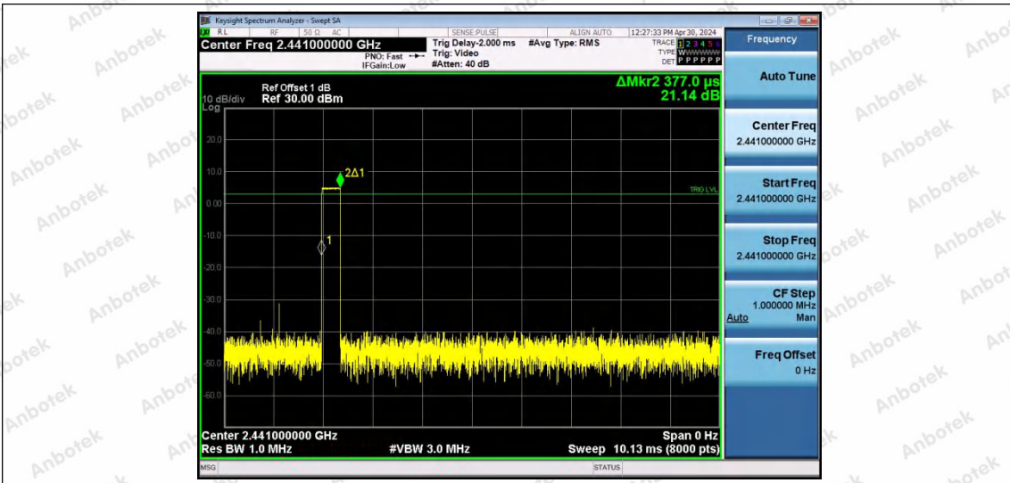
DH1-Ant0-Hop-PASS
