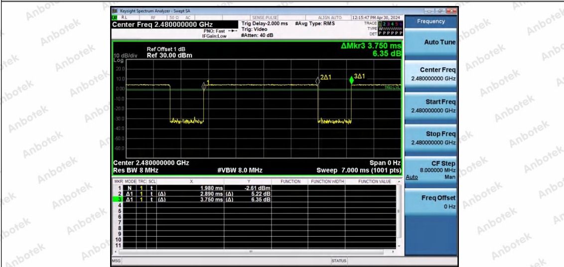
NTNV-3DH5-Ant0-2480
