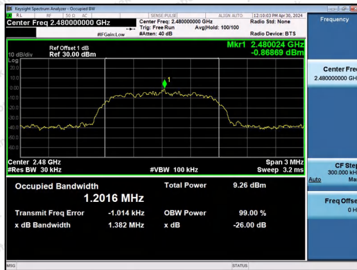
2DH5-Ant0-2480
