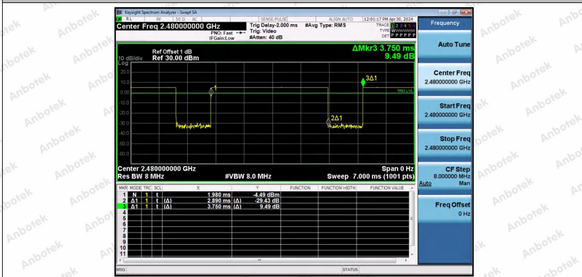
NTNV-DH5-Ant0-2480
