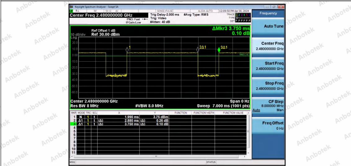
NTNV-2DH5-Ant0-2480
