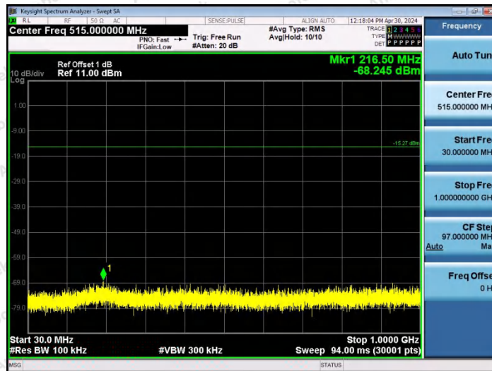
DH5-Ant0-2402-30~1000-PASS
