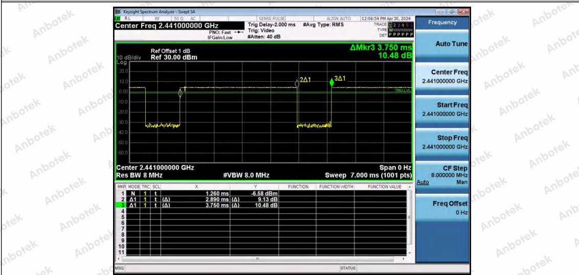
NTNV-2DH5-Ant0-2441
