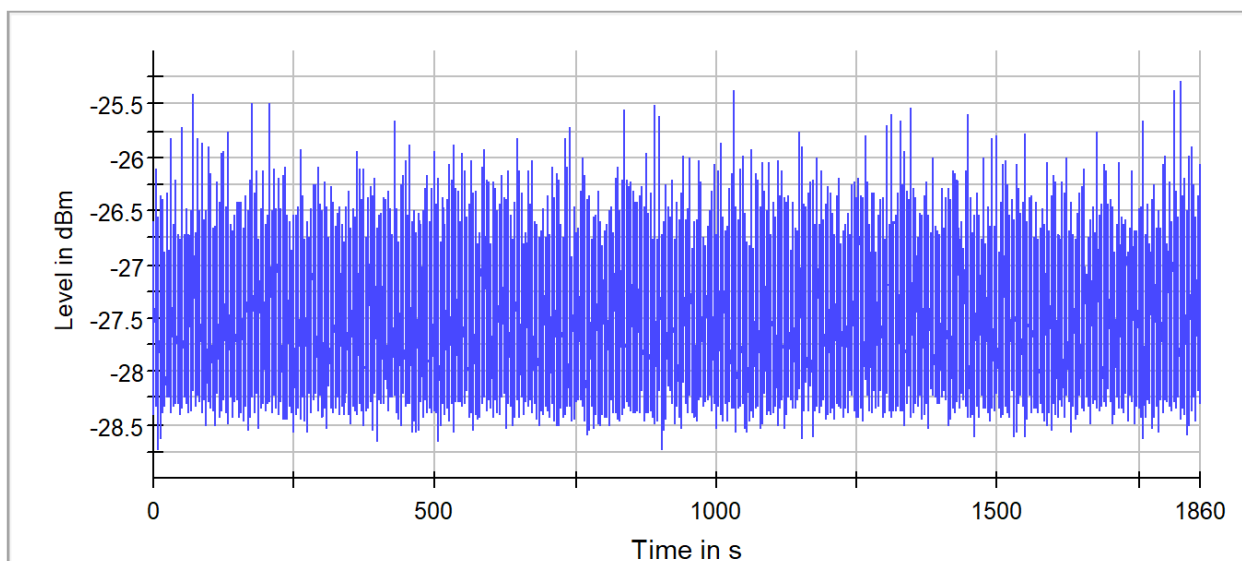
802.11ac(40 MHz) Channel 54
