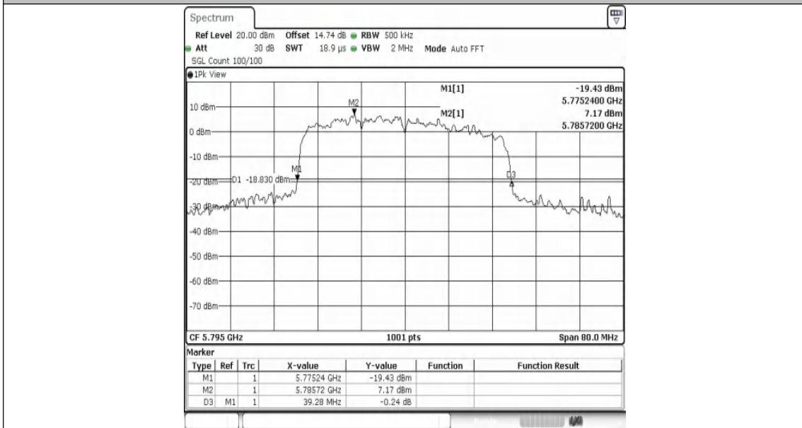
11AX40MIMO-Ant1-5795
