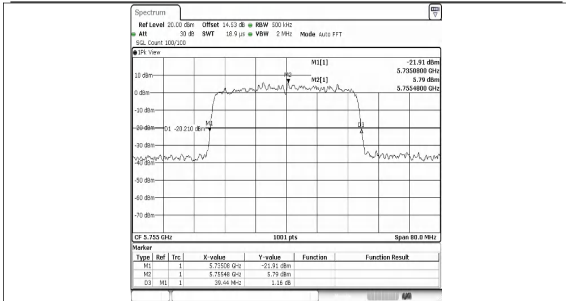
11AX40MIMO-Ant1-5755
