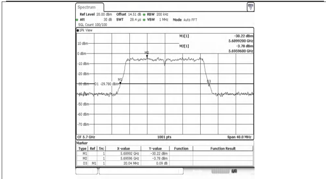
11N20MIMO-Ant1-5700
