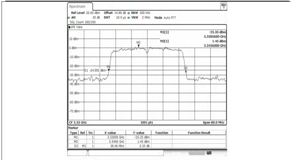
11AC40MIMO-Ant1-5550
