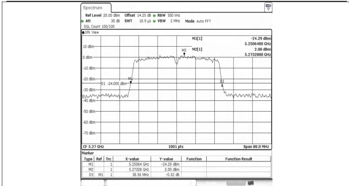
11AC40MIMO-Ant1-5270
