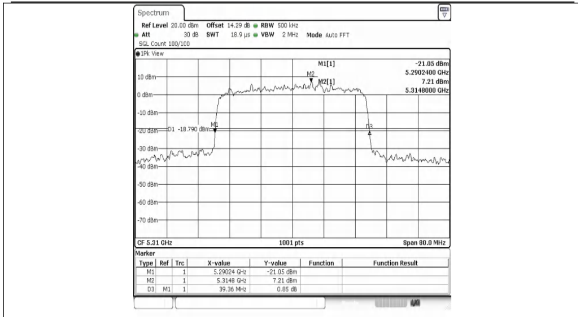
11AX40MIMO-Ant1-5310
