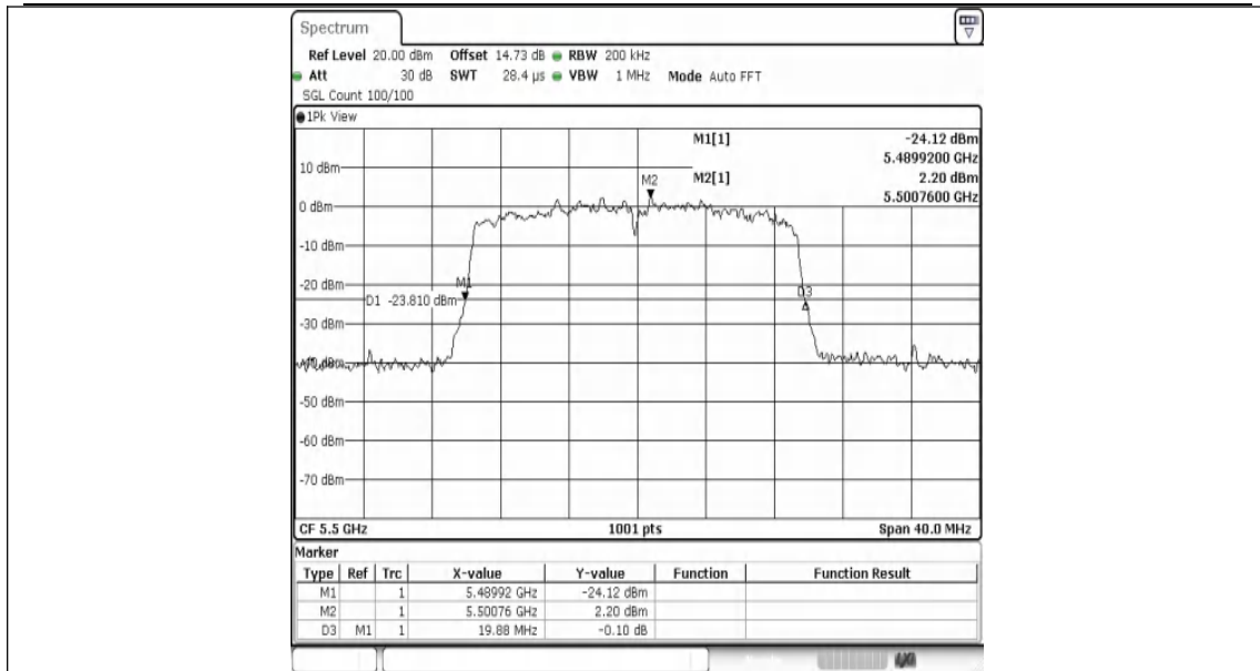
11AX20MIMO-Ant1-5500
