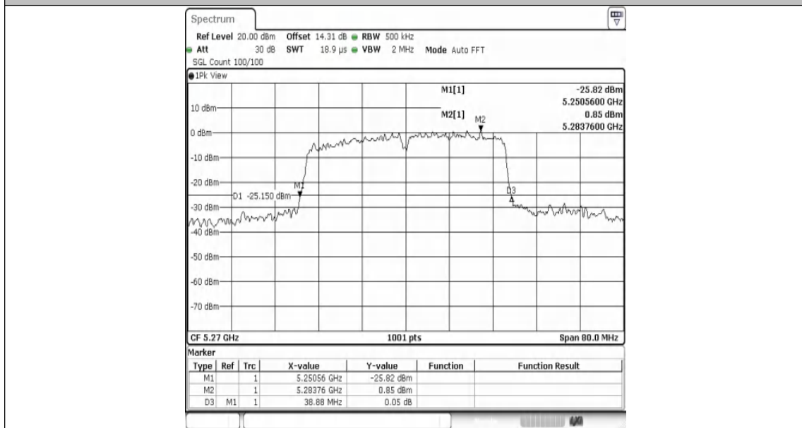
11AC40MIMO-Ant1-5270
