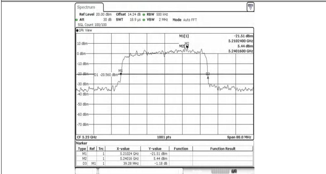
11AX40MIMO-Ant1-5230
