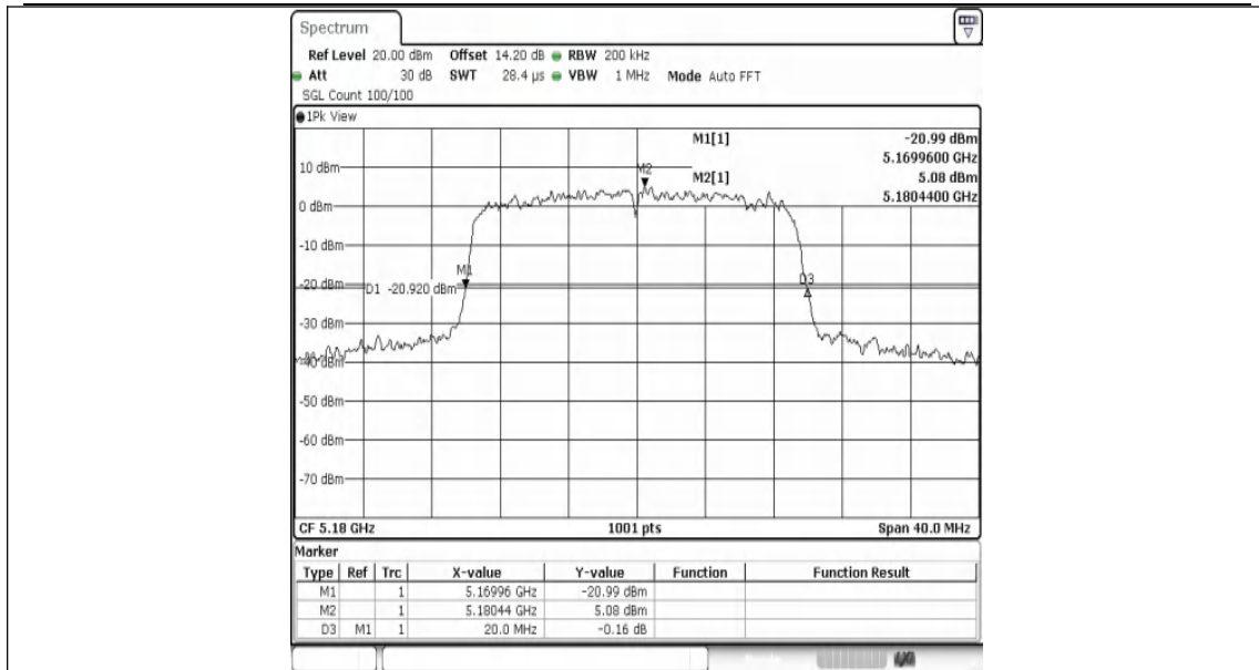
11AX20MIMO-Ant1-5180
