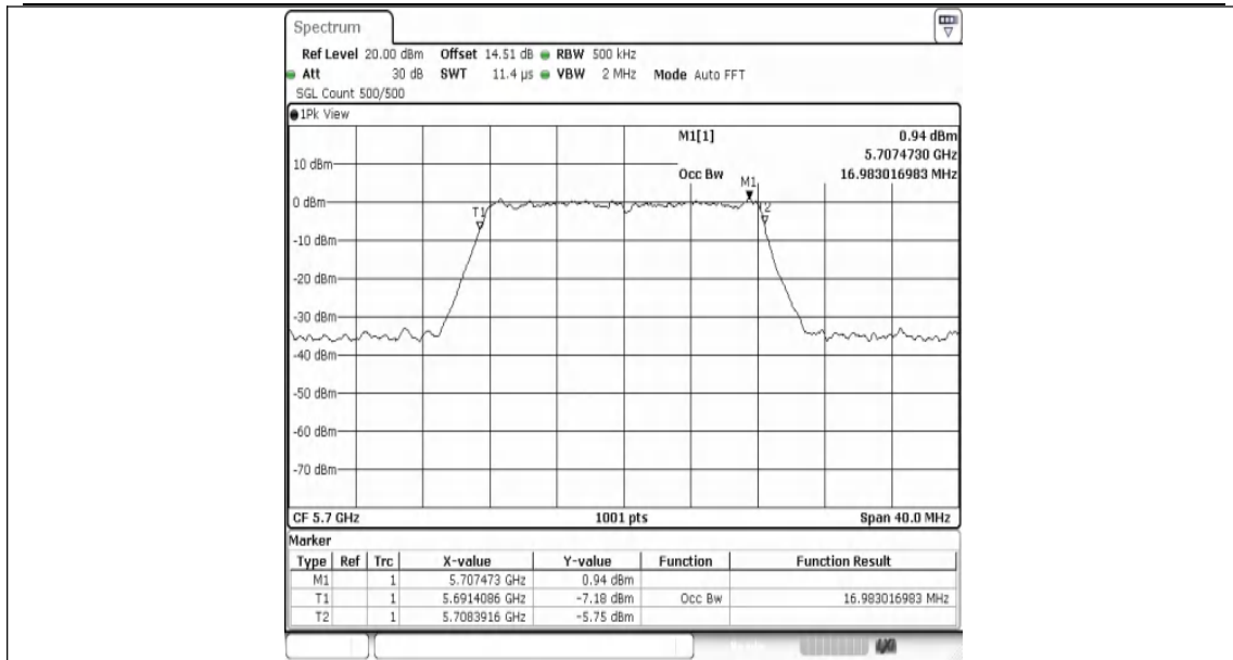
11A-Ant1-5700
