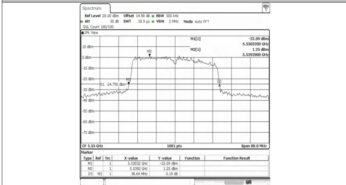
11AC40MIMO-Ant1-5550
