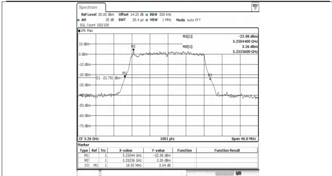
11A-Ant1-5260
