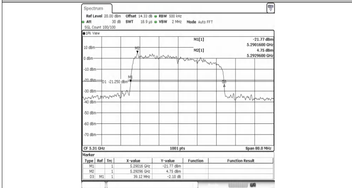
11AX40MIMO-Ant1-5310
