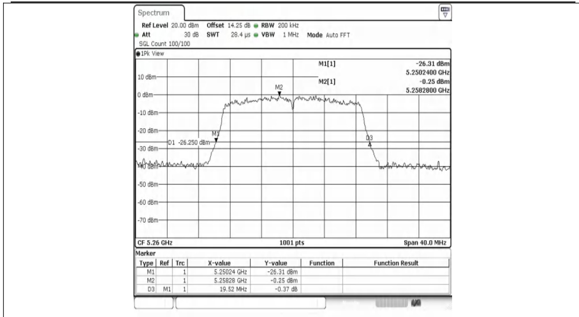
11AC20MIMO-Ant1-5260
