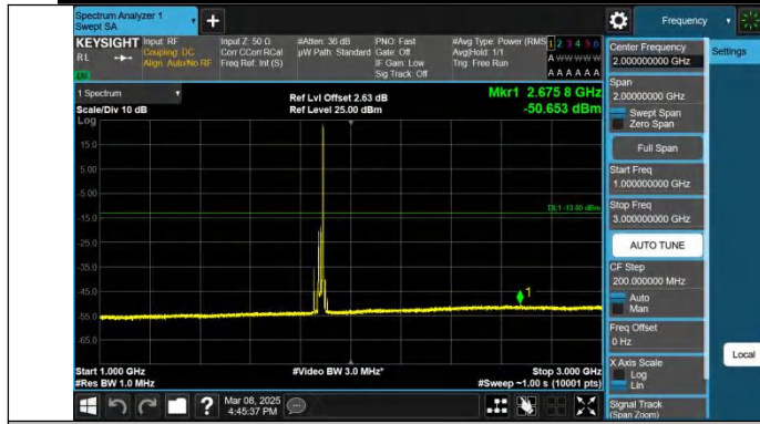
Band2-20MHz-QPSK-18900-1RB#99-1000~3000-PASS
