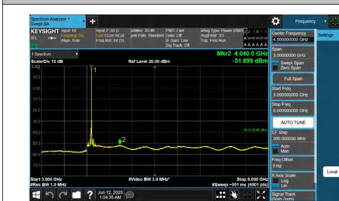
48-48-20MHz-20MHz-QPSK-QPSK-56442-56640-1RB#0-0RB#0- 3000~6000MHz-PASS
