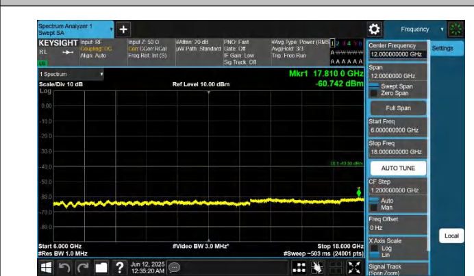
48-48-20MHz-20MHz-QPSK-QPSK-56442-56640-1RB#0-0RB#0- 6000~18000MHz-PASS
