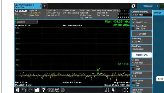
48-48-20MHz-20MHz-QPSK-QPSK-56442-56640-1RB#99-0RB# 0-0.009~0.15MHz-PASS
