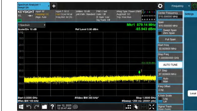
48-48-20MHz-20MHz-QPSK-QPSK-56442-56640-1RB#99-0RB# 0-30~1000MHz-PASS
