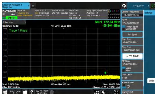
NTNV-n48-PC3-30-20-L-DFT-QPSK-Inner_1RB_Left-30-1000-PA SS
