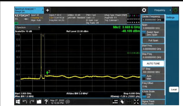
42-42-20MHz-15MHz-QPSK-QPSK-42841-43012-1RB#0-0RB#0- 3000~6000MHz-PASS
