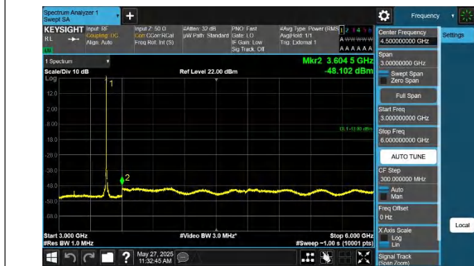
42-42-20MHz-20MHz-QPSK-QPSK-42190-42388-1RB#0-0RB#0- 3000~6000MHz-PASS
