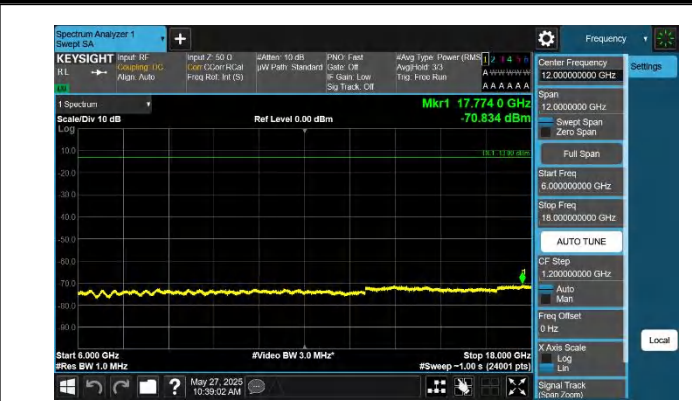
42-42-20MHz-10MHz-QPSK-QPSK-42891-43035-1RB#99-0RB# 0-6000~18000MHz-PASS
