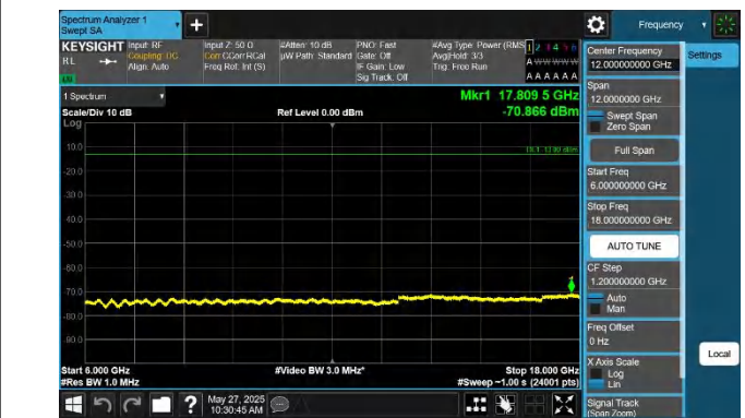
42-42-20MHz-10MHz-QPSK-QPSK-42190-42334-1RB#0-0RB#0- 6000~18000MHz-PASS
