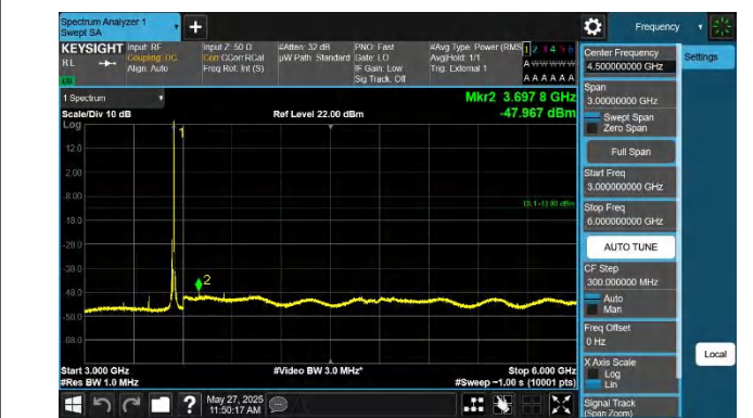
42-42-20MHz-5MHz-QPSK-QPSK-42940-43057-1RB#99-0RB#0- 3000~6000MHz-PASS
