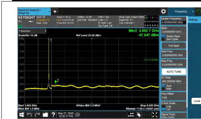
42-42-20MHz-10MHz-QPSK-QPSK-42891-43035-1RB#99-0RB# 0-3000~6000MHz-PASS
