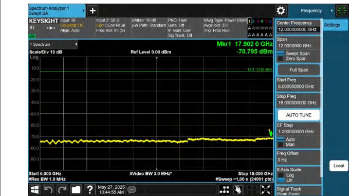
42-42-20MHz-15MHz-QPSK-QPSK-42516-42687-1RB#0-0RB#0- 6000~18000MHz-PASS
