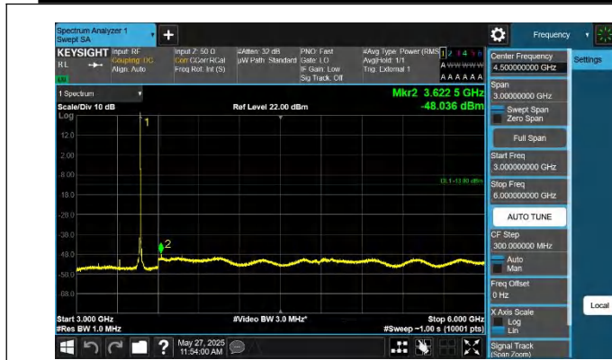
42-42-20MHz-10MHz-QPSK-QPSK-42190-42334-1RB#99-0RB# 0-3000~6000MHz-PASS
