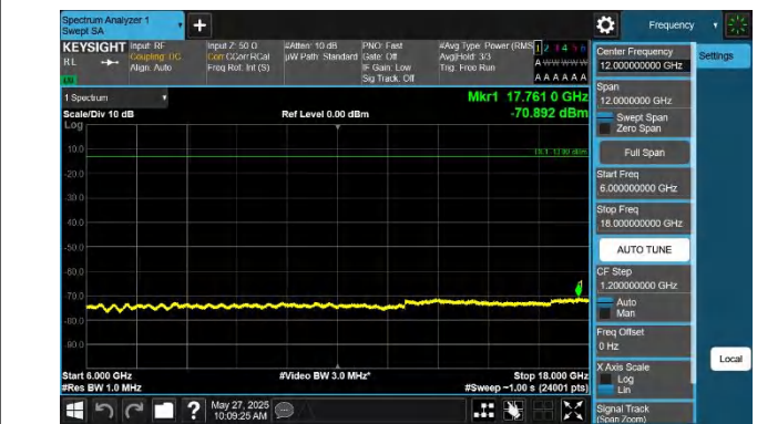
42-42-20MHz-20MHz-QPSK-QPSK-42190-42388-1RB#0-0RB#0- 6000~18000MHz-PASS
