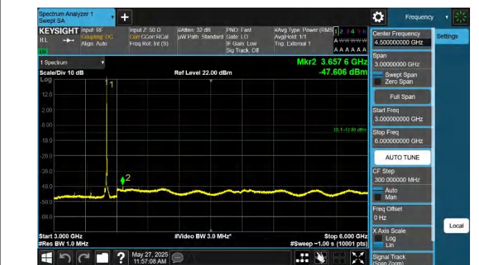
42-42-20MHz-10MHz-QPSK-QPSK-42541-42685-1RB#99-0RB# 0-3000~6000MHz-PASS
