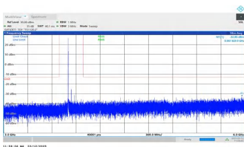
NTNV-n77(3700-3980)-PC2-30-80-M-DFT-QPSK-Inner_1RB_Lef t-3000-6000-PASS
