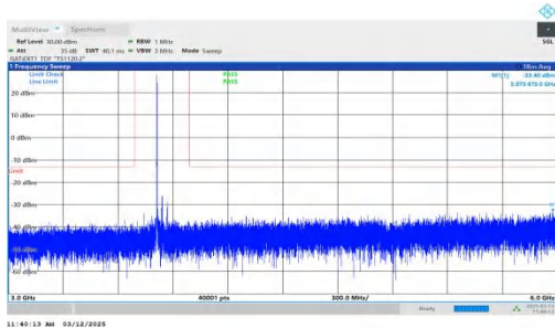
NTNV-n77(3700-3980)-PC2-30-60-M-DFT-QPSK-Inner_1RB_Lef t-3000-6000-PASS
