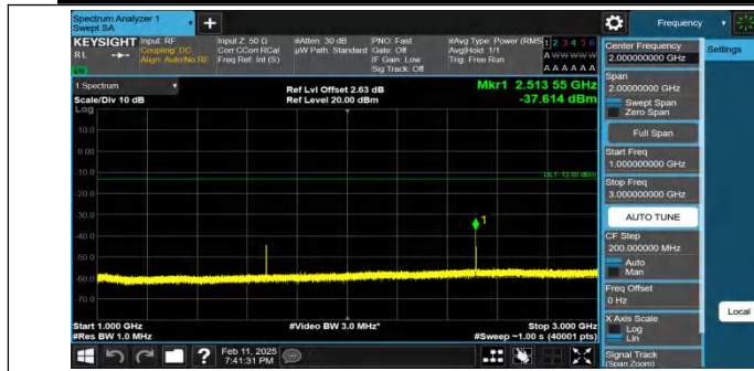
Band26(824-849)-3MHz-QPSK-26915-1RB#14-1000~3000-PASS
