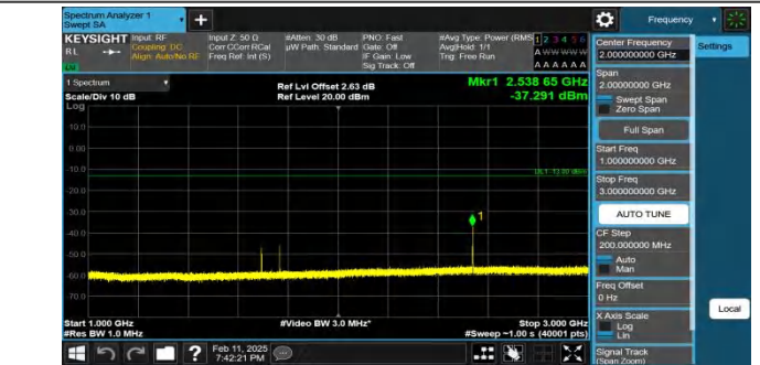
Band26(824-849)-3MHz-QPSK-27025-1RB#0-1000~3000-PASS
