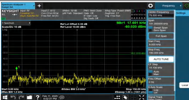
Band26(824-849)-10MHz-QPSK-26990-1RB#0-0.009~0.15-PASS
