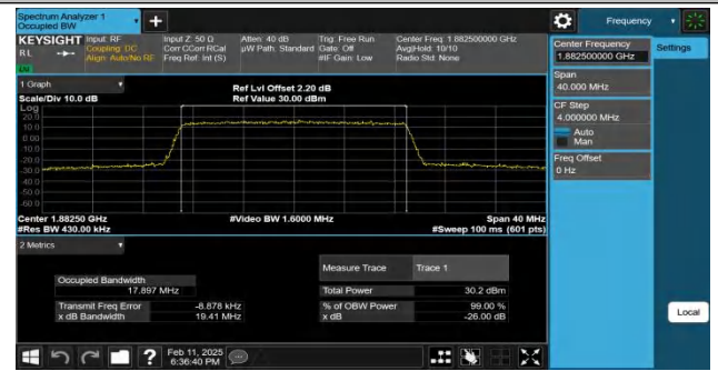
Band25-20MHz-16QAM-26365-100RB#0-PASS
