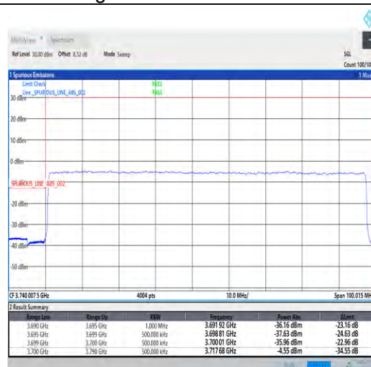
1-N78-3700-3800-30-90-L-3-DFT-PI2BPSK-Outer _Full-240@0-Ant0-1--PASS-see graph
