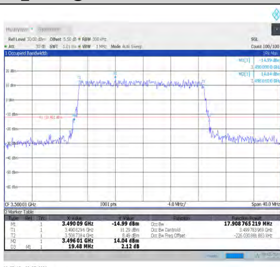
1-N78-3450-3550-PC2-30-20-M-5-DFT-256QAM-Out er_Full-50@0-Ant0-17.909-19.480-≤20-PASS
