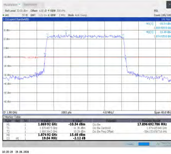
1-N2-15-20-M-2-DFT-PI2BPSK-Outer_Full-100@0-A nt0-17.897-19.040-≤20-PASS
