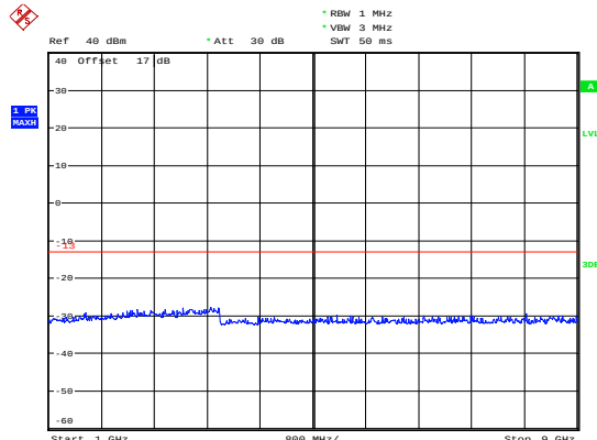
GSM 850 CH-Low 1GHz ~ 9GHz
