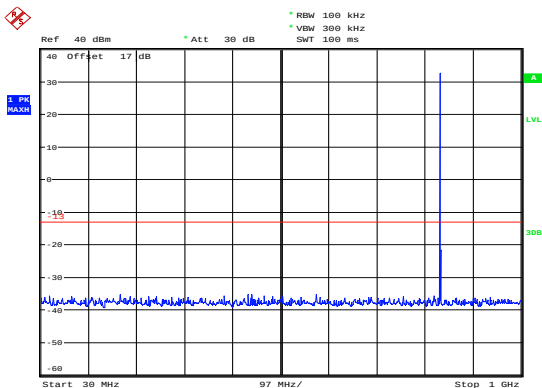
GSM 850 CH- Middle 30MHz ~ 1GHz
