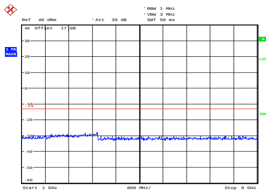
GSM 850 CH- Middle 1GHz ~ 9GHz
