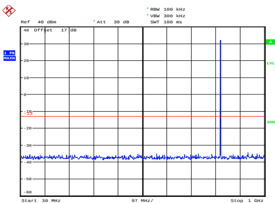
GSM 850 CH-Low 30MHz ~ 1GHz
