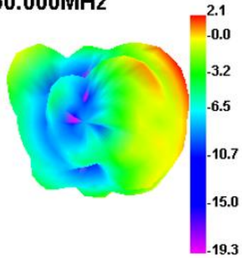
2450.000MHz
