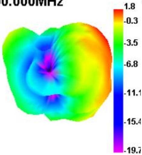
2500.000MHz
