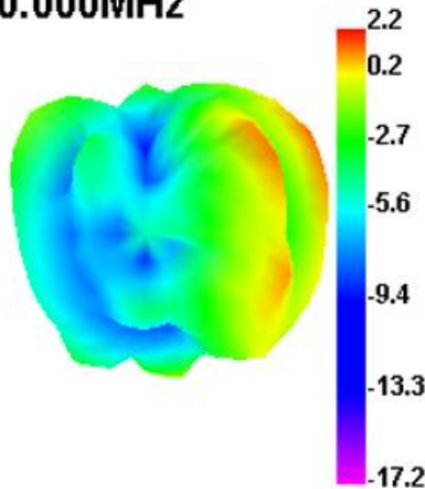
2500.000MHz
