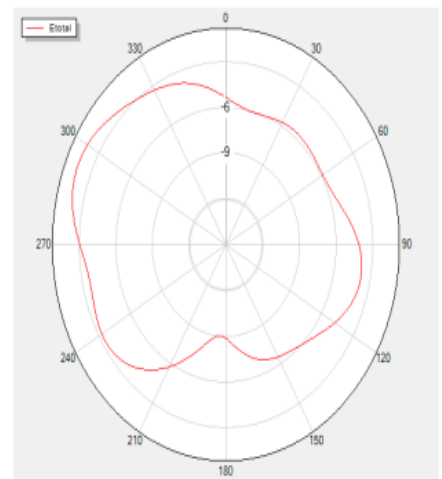
Theta=90 Freq=2420MHz
