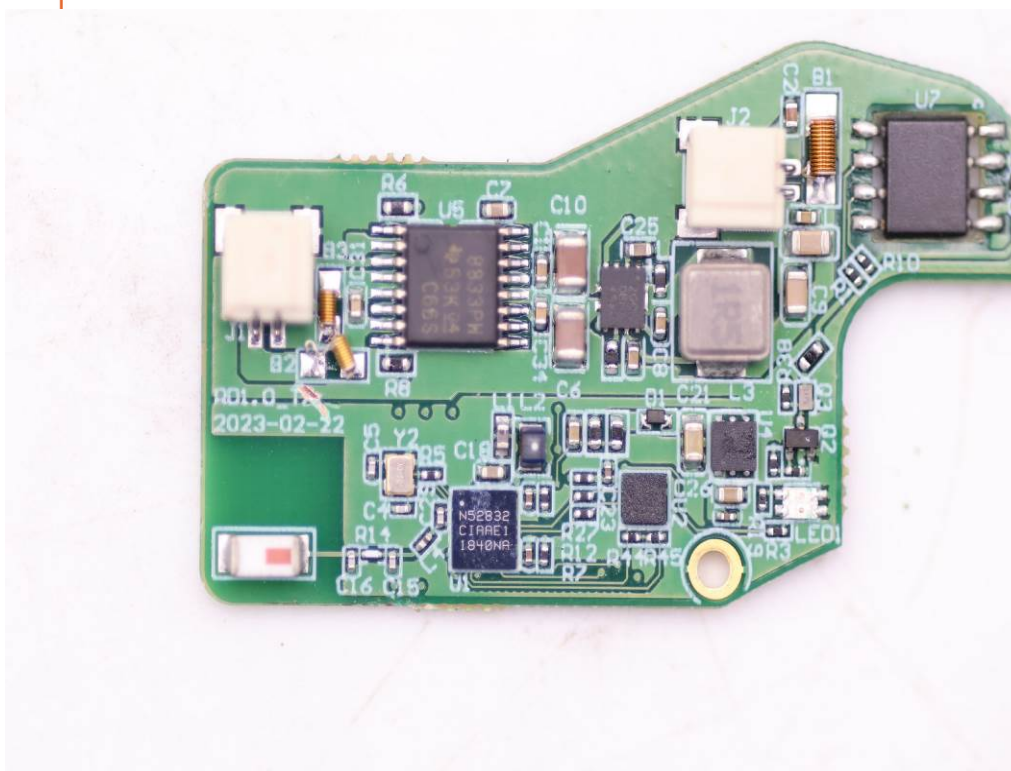
Antenna
