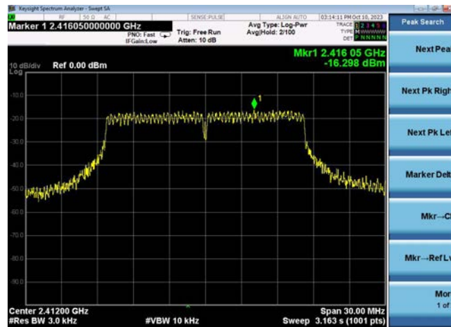
CH01
