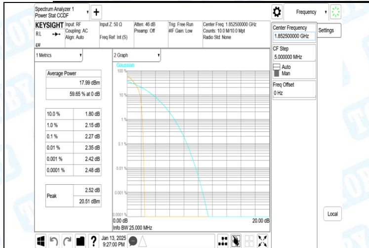
Band2-5MHz-QPSK-18625-1RB#0-PASS
