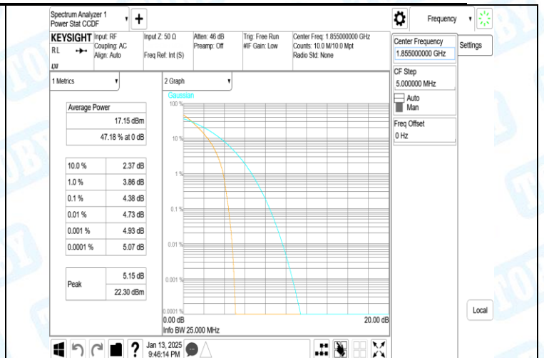
Band2-10MHz-QPSK-18650-50RB#0-PASS
