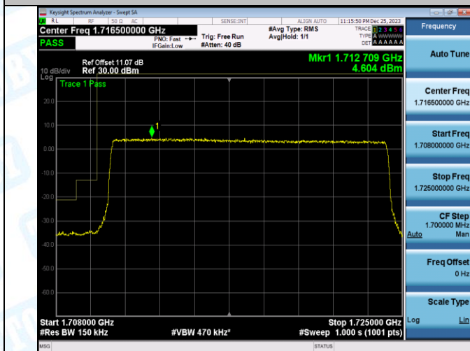
Band4_15MHz_QPSK_2025_1RB#0
