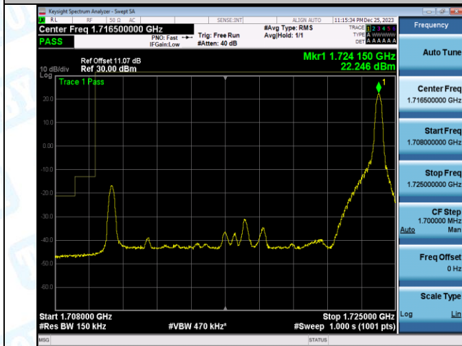
Band4_15MHz_QPSK_2025_75RB#0
