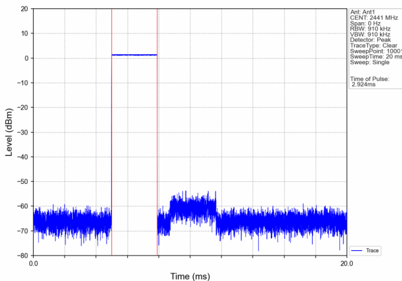
GFSK_DH5_HOPP_Ant1_NTNV
