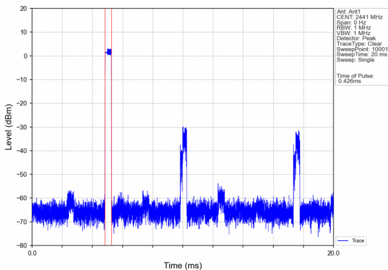
Pi/4DQPSK_2DH1_HOPP_Ant1_NTNV
