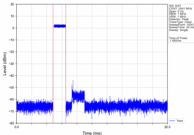
Pi/4DQPSK_2DH3_HOPP_Ant1_NTNV
