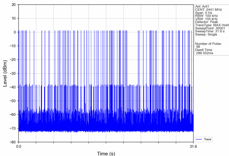
GFSK_DH5_HOPP_Ant1_NTNV
