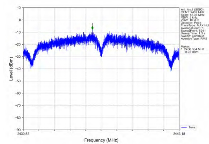
802.11b_MCH_2437MHz_Ant1 (SISO)_NTNV
