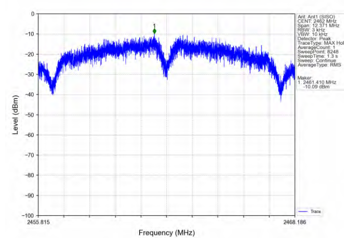
802.11b_HCH_2462MHz_Ant1 (SISO)_NTNV
