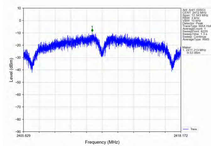
802.11b_LCH_2412MHz_Ant1 (SISO)_NTNV
