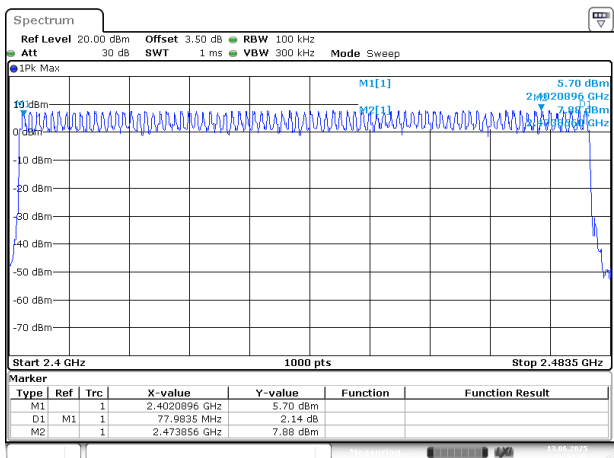
EDR(8DPSK)_3DH1_Hopping
