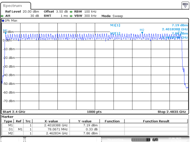
EDR( \pi/4 -DQPSK)_2DH1_Hopping
