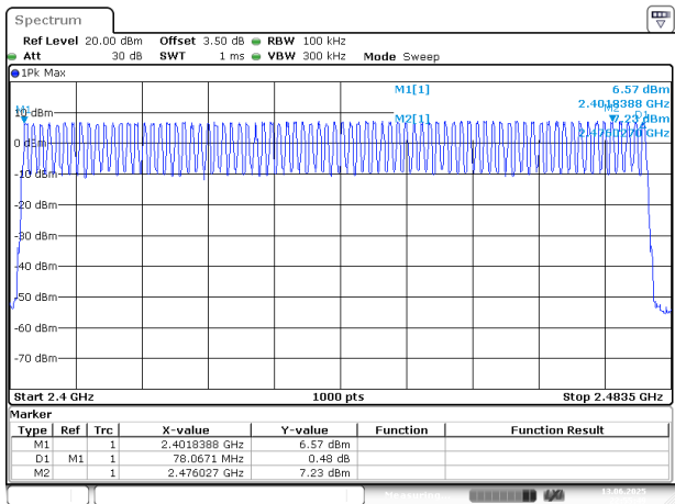
BDR(GFSK)_DH1_Hopping
