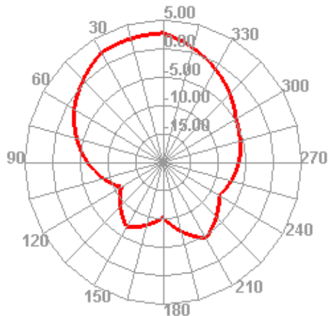
2450.000MHz E1
