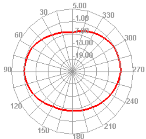
2450.000MHz H
