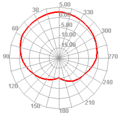
2450.000MHz E2
