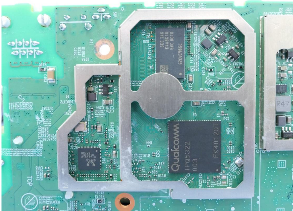
(8) EUT Photo
