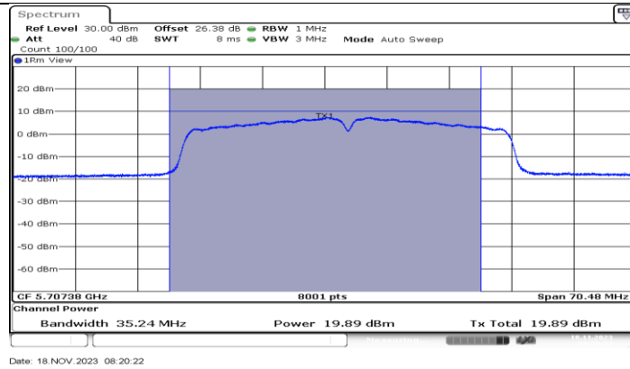
11N40MIMO_Ant1_5710_UNII-2C
