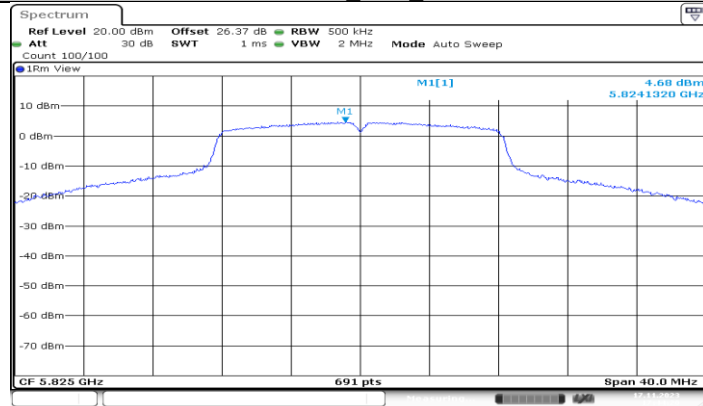
11A-CDD_Ant1_5825
