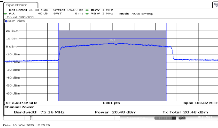
11AX80MIMO_Ant1_5690_UNII-2C
