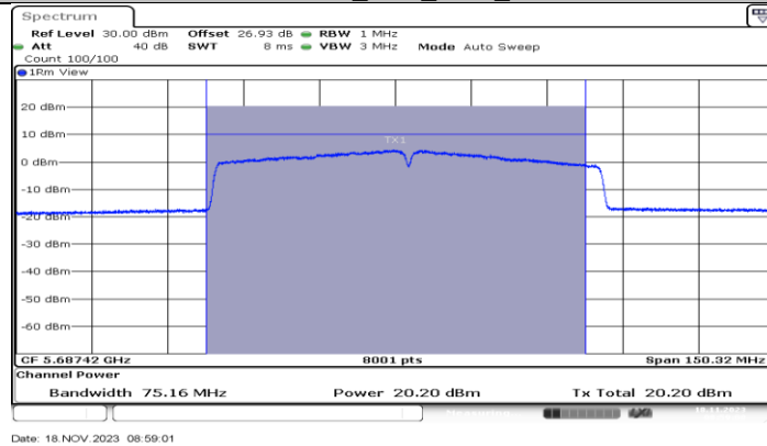
11AC80MIMO_Ant2_5690_UNII-2C
