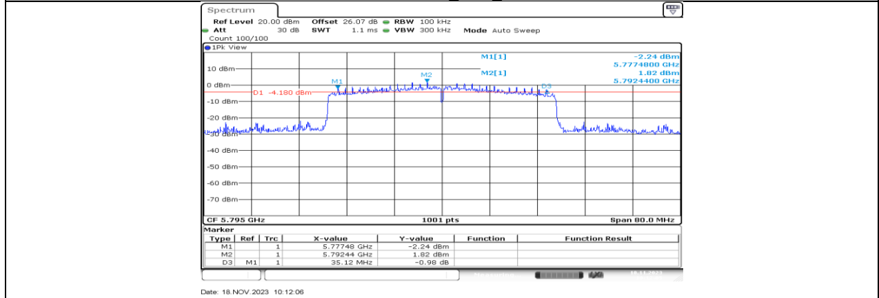
11AX40MIMO_Ant2_5795
