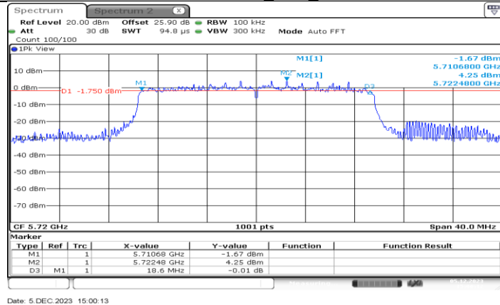
11AX20MIMO_Ant1_5720
