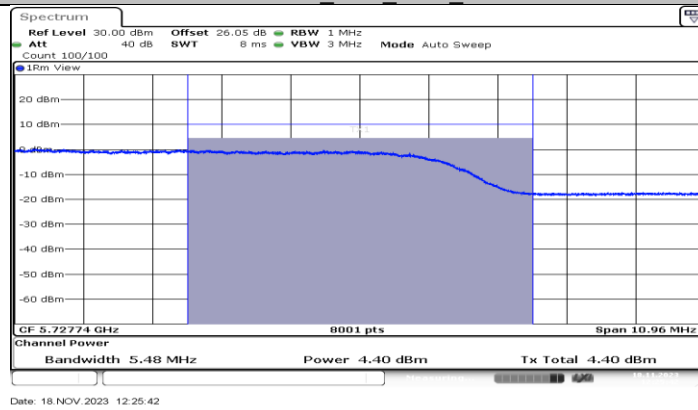
11AX80MIMO_Ant1_5690_UNII-3
