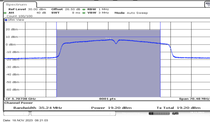
11N40MIMO_Ant2_5710_UNII-2C
