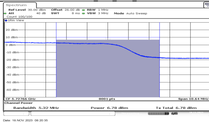
11N40MIMO_Ant1_5710_UNII-3
