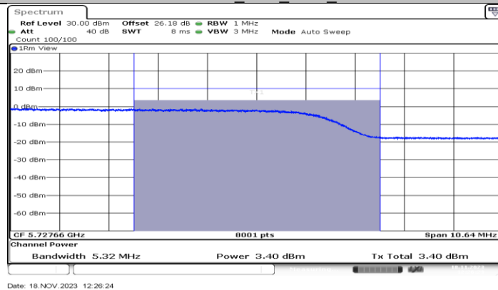
11AX80MIMO_Ant2_5690_UNII-3
