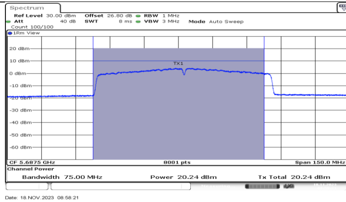
11AC80MIMO_Ant1_5690_UNII-2C
