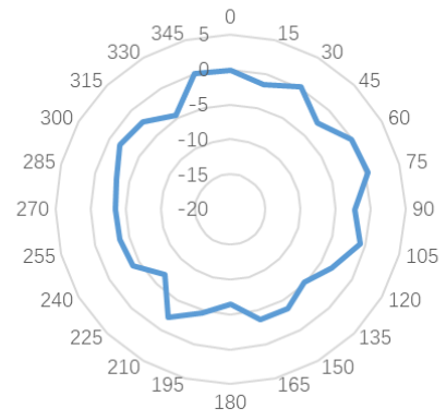
5750MHz_Theta=90°
