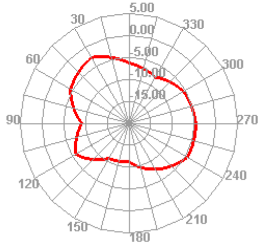
2500.000MHz H
