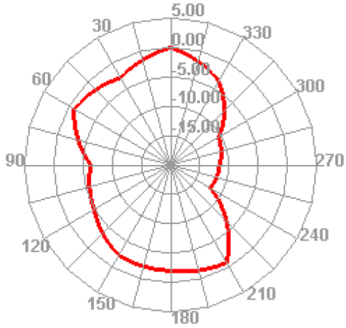
2450.000MHz E1
