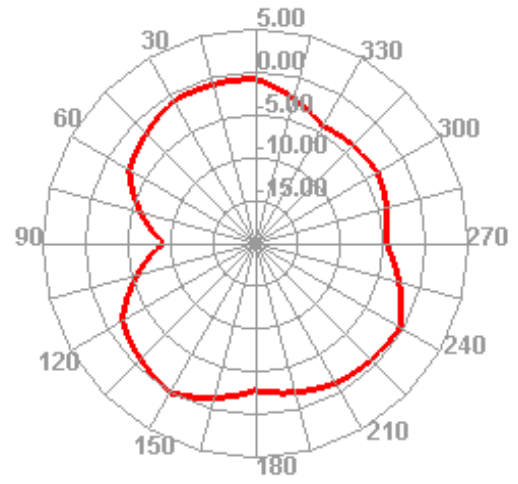
2500.000MHz E2
