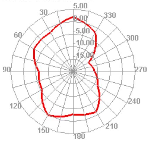
2500.000MHz E1
