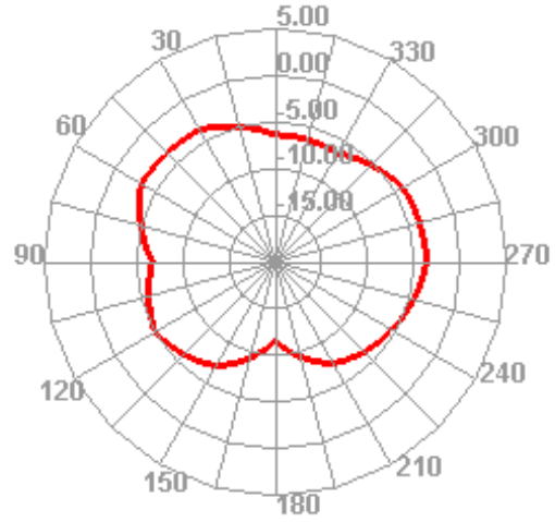
2450.000MHz H
