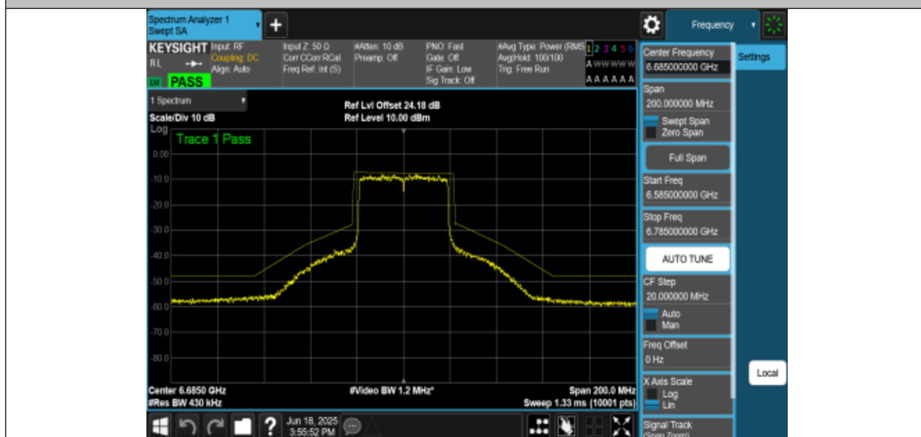
NTNV-11AX40MIMO-Ant1-6685-PASS
