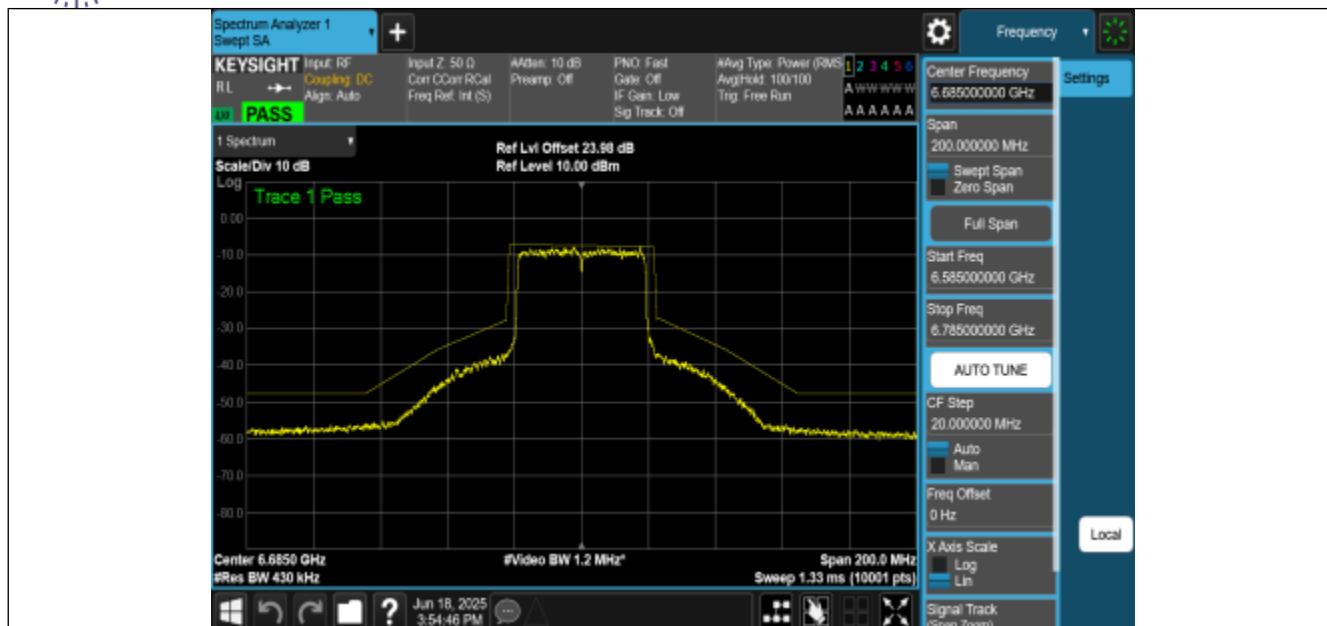
NTNV-11AX40MIMO-Ant0-6685-PASS
