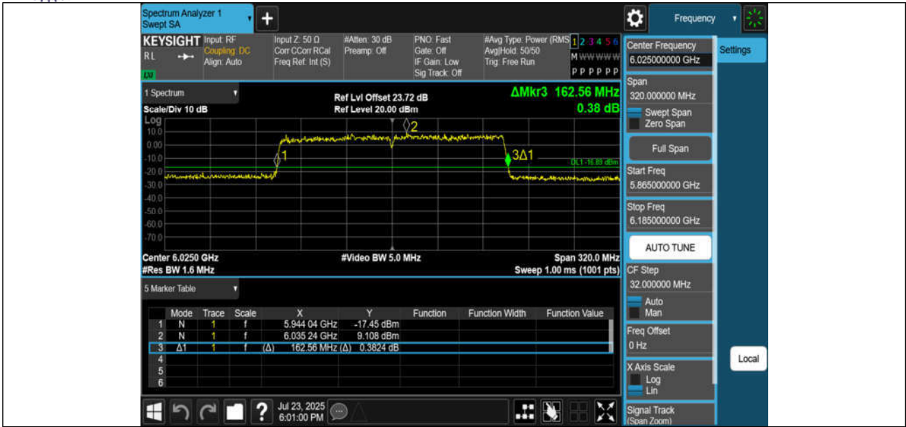
11BE160MIMO-Ant3-6025
