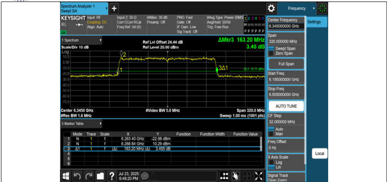
11BE160MIMO-Ant3-6345
