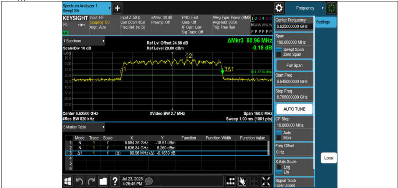
11BE80MIMO-Ant3-6625
