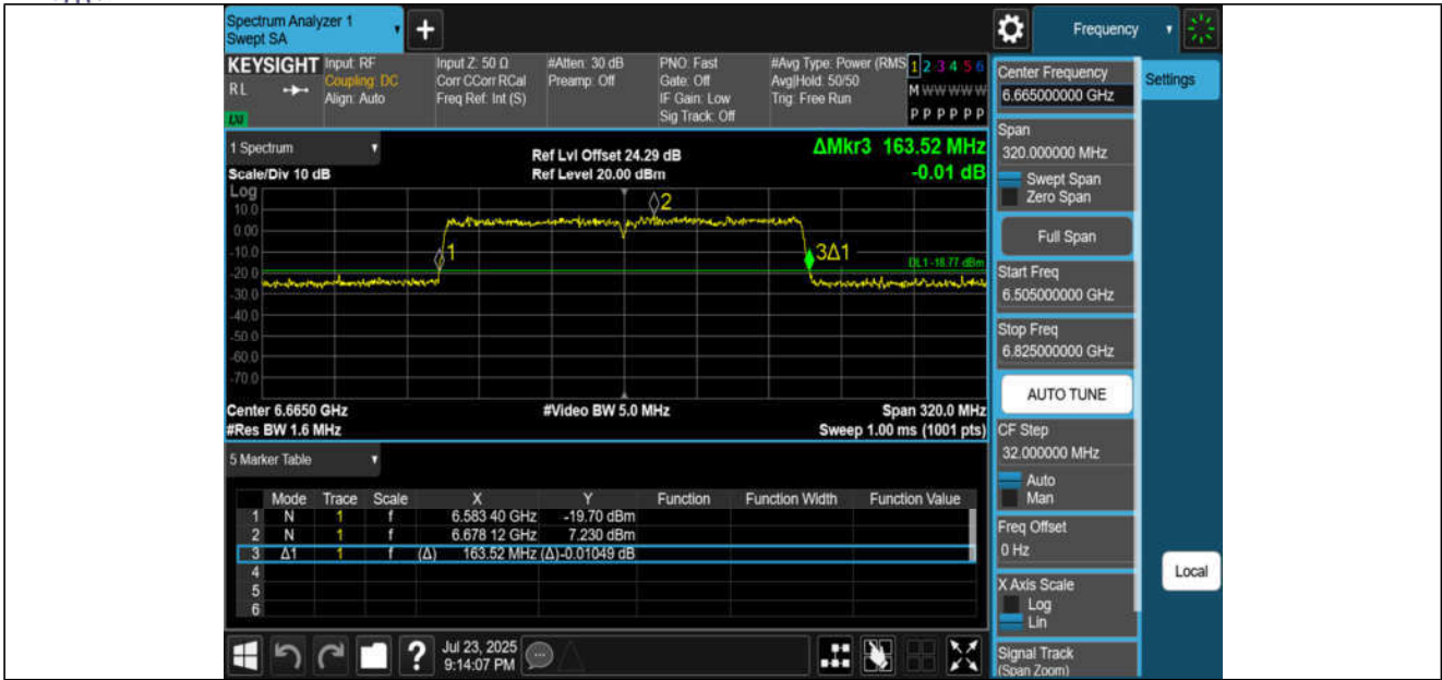
11BE160MIMO-Ant1-6665
