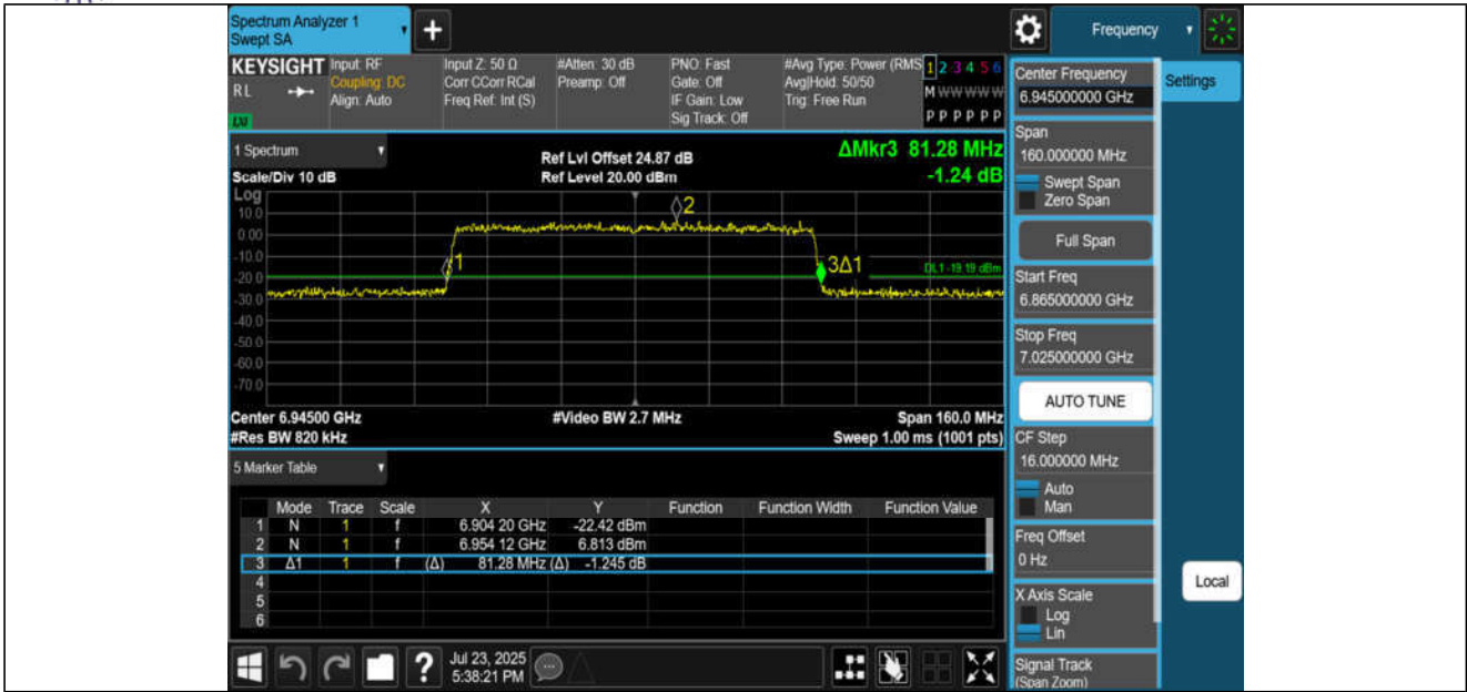
11BE80MIMO-Ant3-6945
