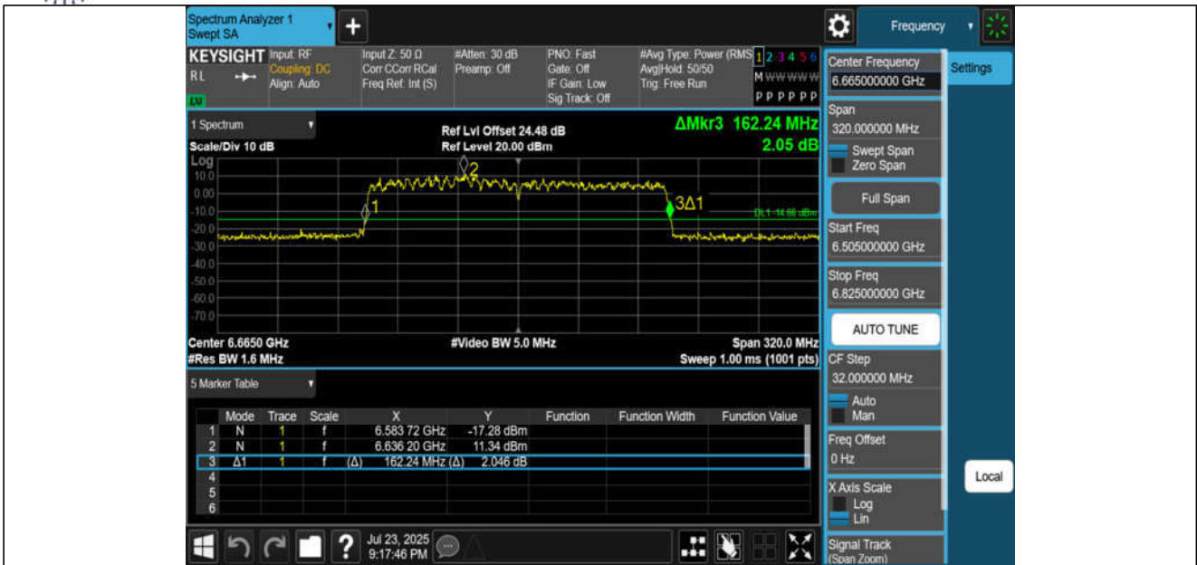
11BE160MIMO-Ant3-6665
