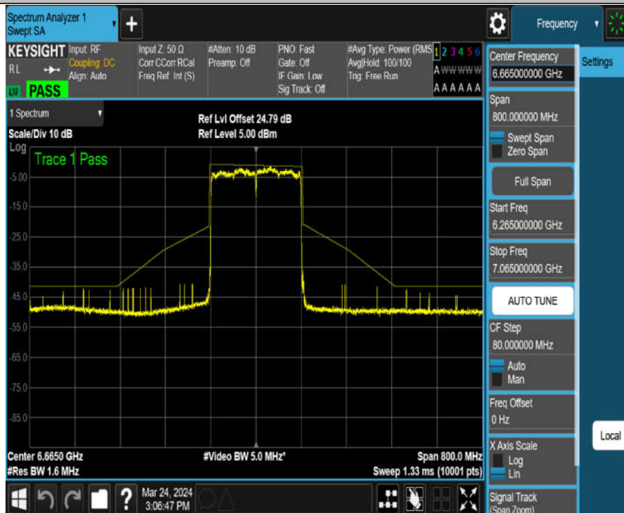
11AX160MIMO_Ant2_6665
