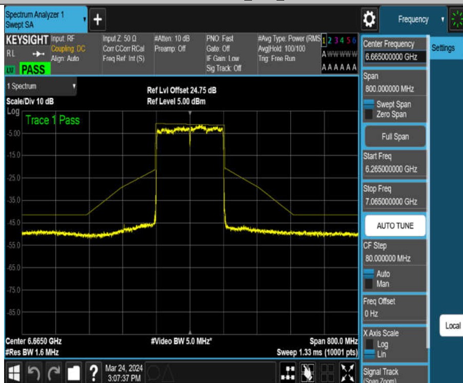
11AX160MIMO_Ant2_6665
