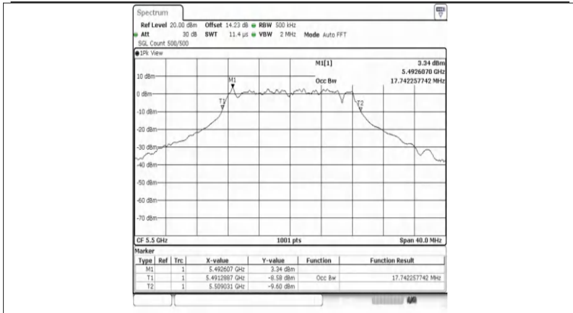
11A-Ant1-5500
