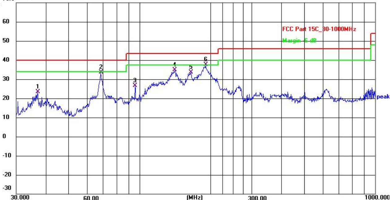
Horizontal dBuV/m
