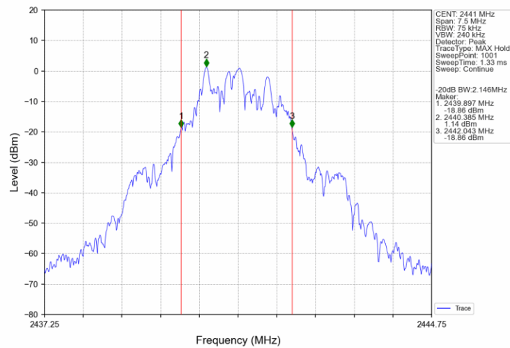
1_MCH_2441MHz_Ant1_NTNV
