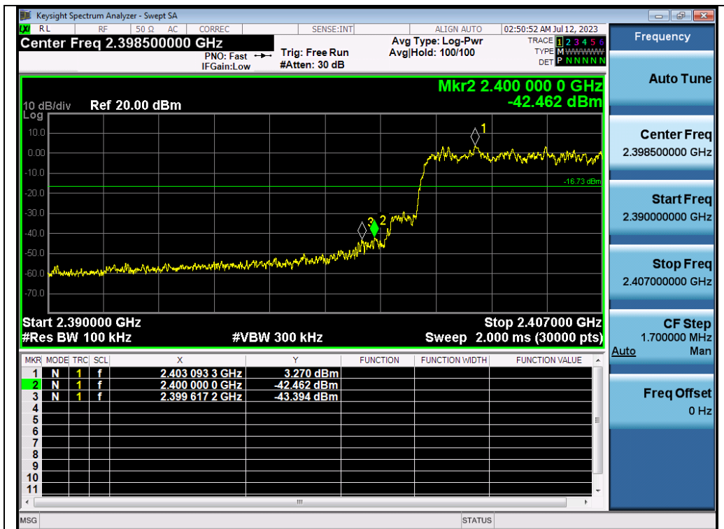
Test_Graph_BR_HOP_ANT1_NA_2Mbps_Lower Band Edge Emissions
