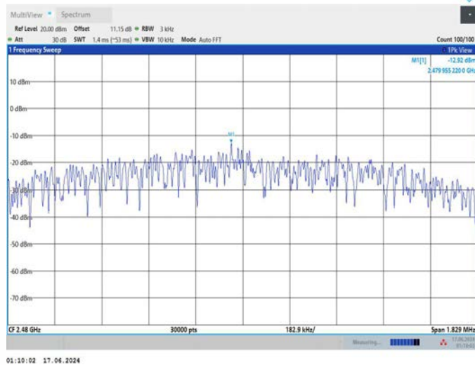
BLE_2M_Ant1_2480
