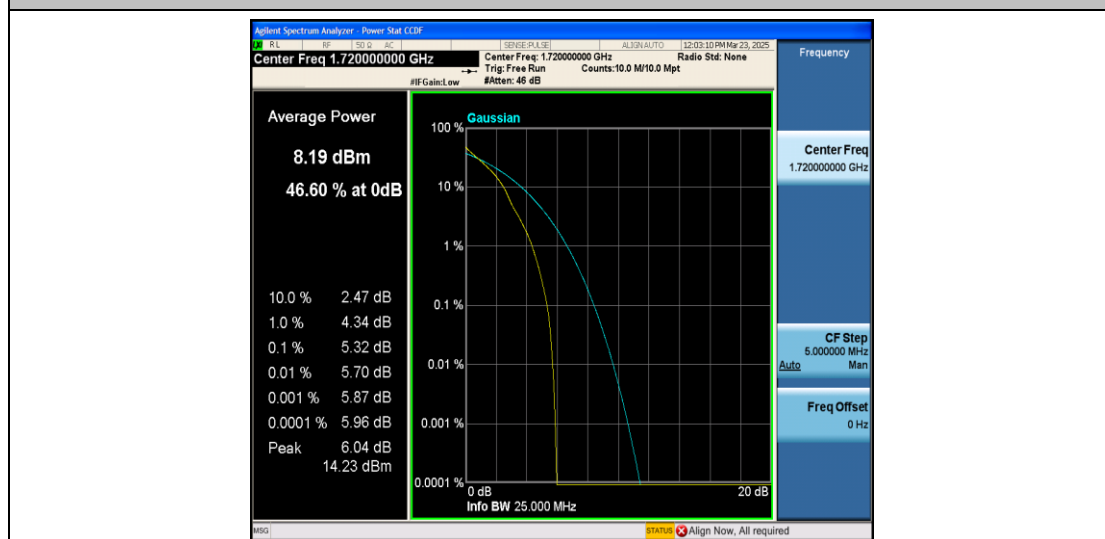
Band66-20MHz-QPSK-132072-1RB#0-PASS
