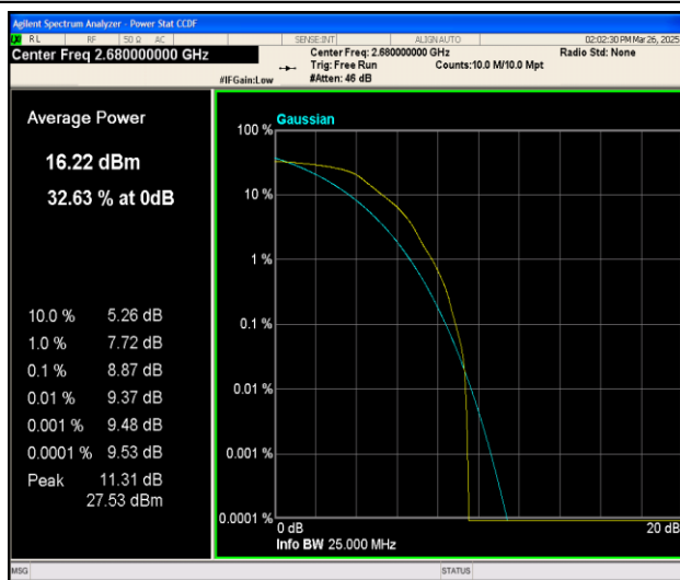
Band41-20MHz-QPSK-41490-1RB#0-PASS
